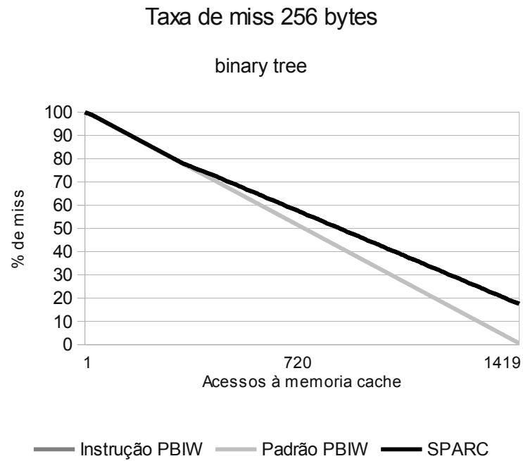
Figura 5.11: Comportamento do programa binary_tree quanto à ocorrência de misses nas caches de instruções e padrões.
