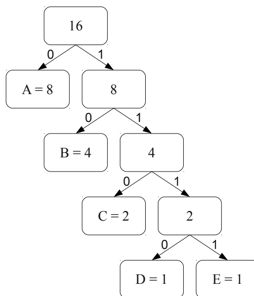
Figura 2.1: Exemplo de árvore de Huffman para a cadeia AAAAAAABBBBBCCDE [1].
