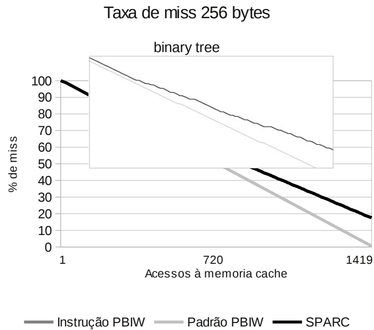
Figura 5.12: Ampliação de trecho do traço de acessos a memória da Figura 5.11.
