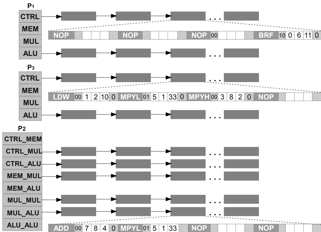
Figura 3.2: Categorias de padrões para o conjunto de instruções VEX [10].
