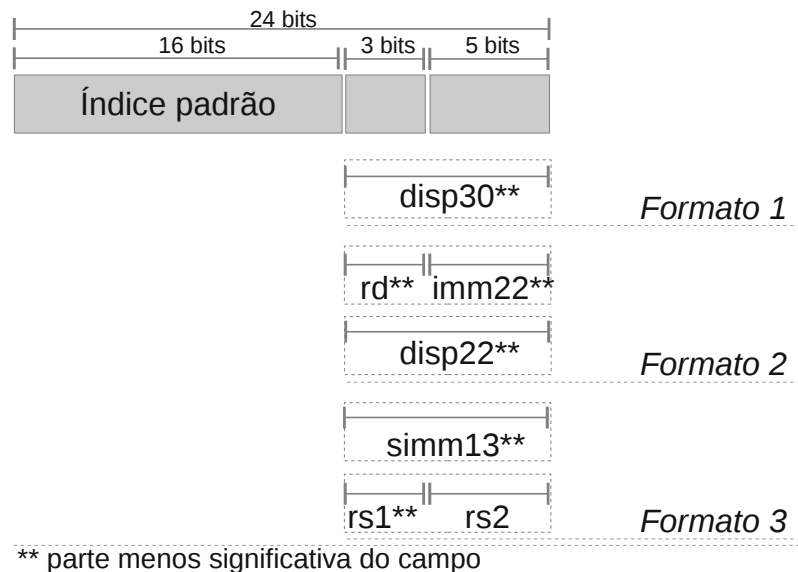
Figura 4.12: Leiaute de instrução PBIW-SPARC de 24 bits.
