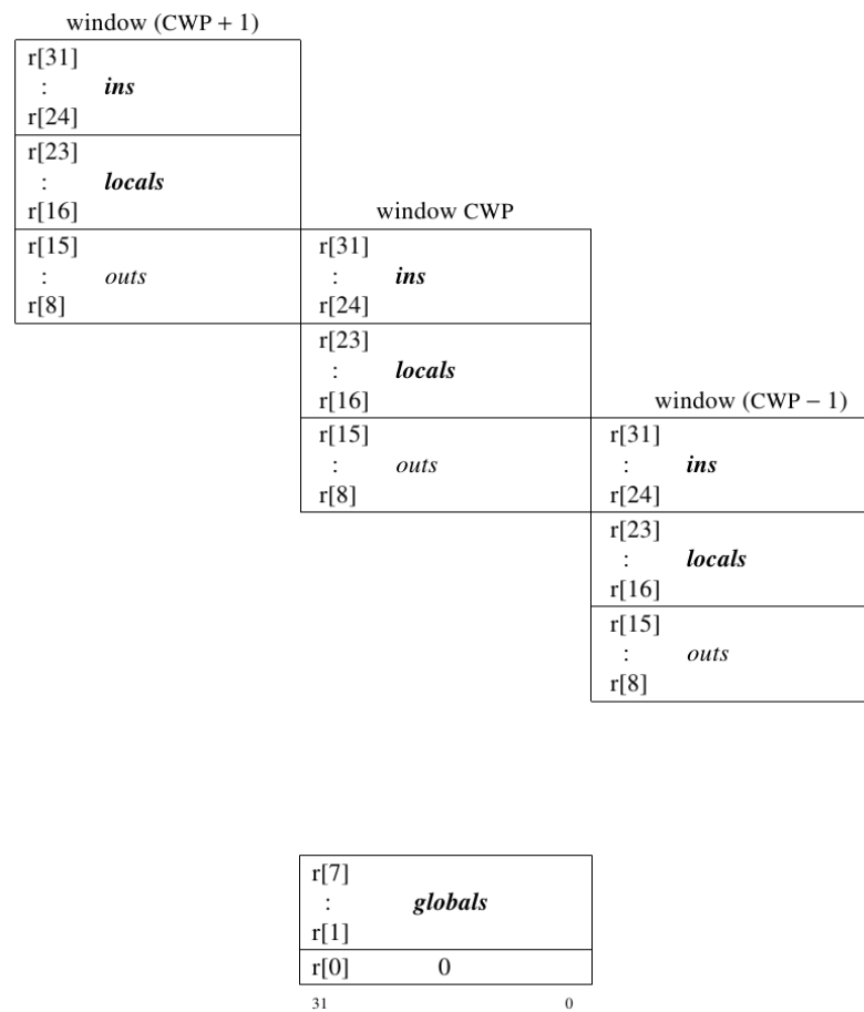
Figura 4.1: Sobreposição das três janelas e os 8 registradores globais [11].
