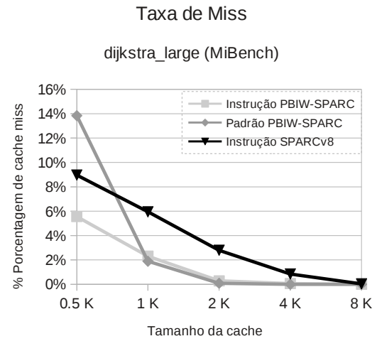
(A.17) dijkstra_large
