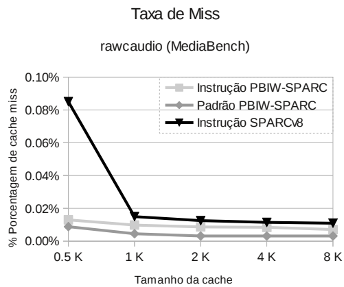
(A.36) rawcaudio
