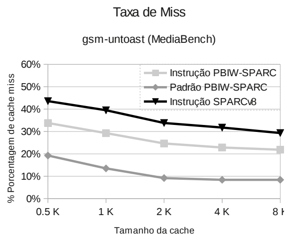
(A.40) untost
