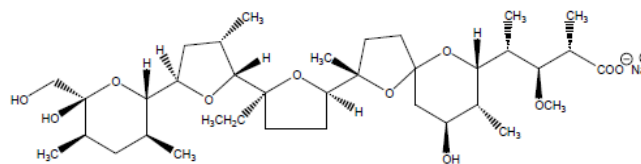
Figura 1. Estrutura molecular da Monensina Na (Page, 2003).
