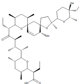
Figura 2. Estrutura molecular da Narasina (Page, 2003).
