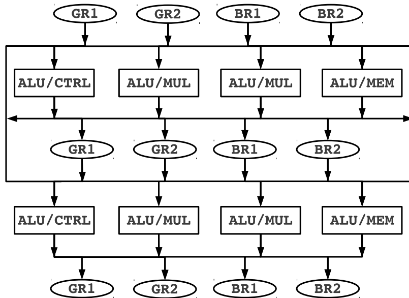
Figura 3.12: Exemplo de desenrolamento do grafo base do \rho -VEX.
