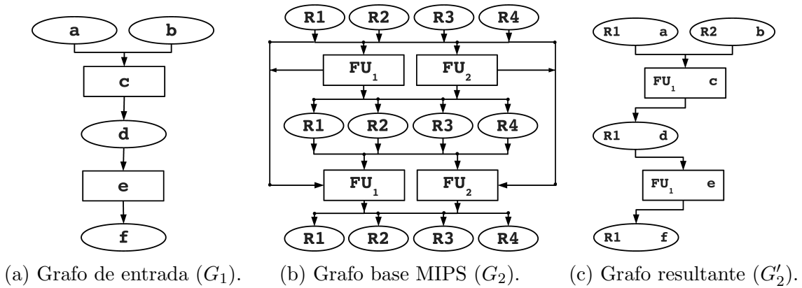
Figura 3.8: Exemplo de Isomorfismo de Subgrafos na arquitetura MIPS.
