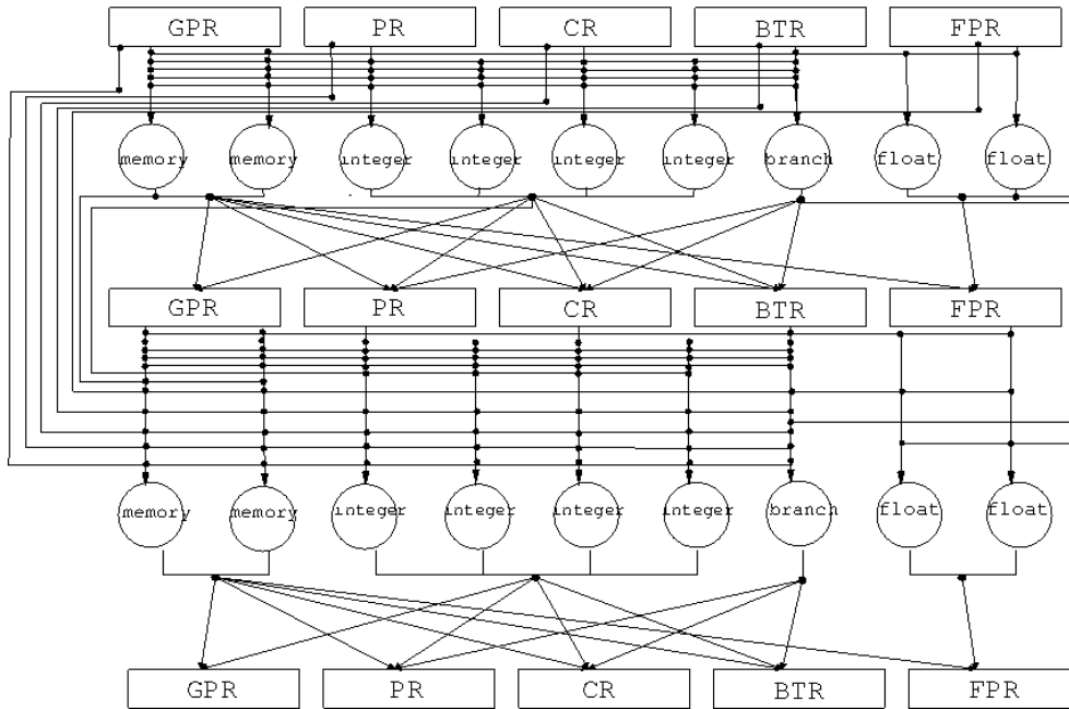
Figura 3.10: Grafo base do processador HPL-PD desenrolado.
