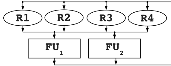
Figura 3.3: Grafo base da arquitetura com duas unidades funcionais e quatro registradores.
