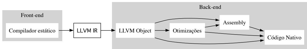
Figura 4.1: Visão em alto nível da infraestrutura LLVM.
