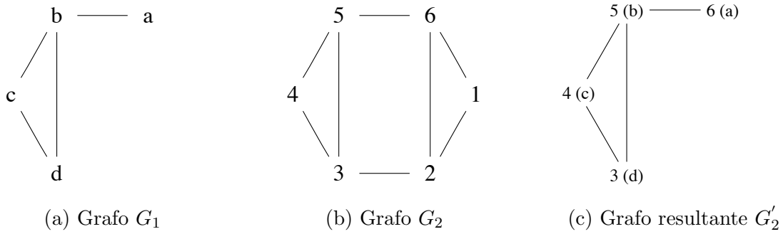
Figura 3.1: Exemplo do problema de isomorfismo de subgrafos.
