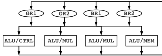
Figura 3.11: Exemplo de grafo base do \rho -VEX.
