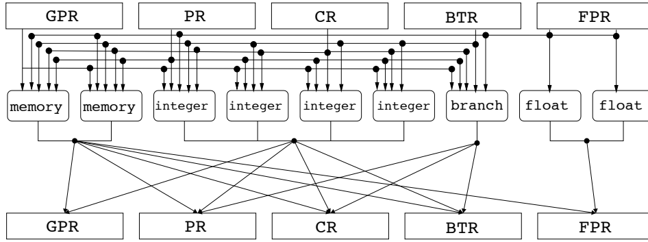
Figura 3.9: Exemplo de grafo base do HPL-PD.
