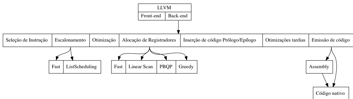
Figura 4.4: Fases do LLVM na geração de código.
