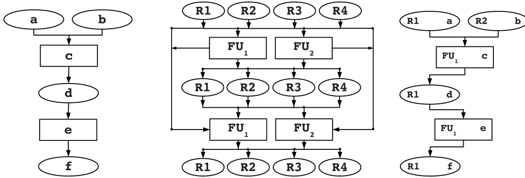
(a) Grafo de entrada ( G_1 ) (b) Grafo base ( G_2 ) com re- (c) Grafo resultante ( G'_2 ) do com operandos explícitos. apresentação de registradores. isomorfismo entre G_1 e G_2 .
