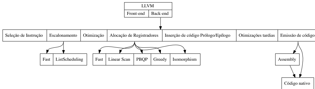
Figura 4.6: Fases do LLVM na geração de código com acréscimo do algoritmo de isomorfismo de subgrafos.
