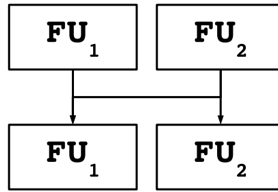
Figura 3.4: Grafo base da arquitetura desenrolado duas vezes.
