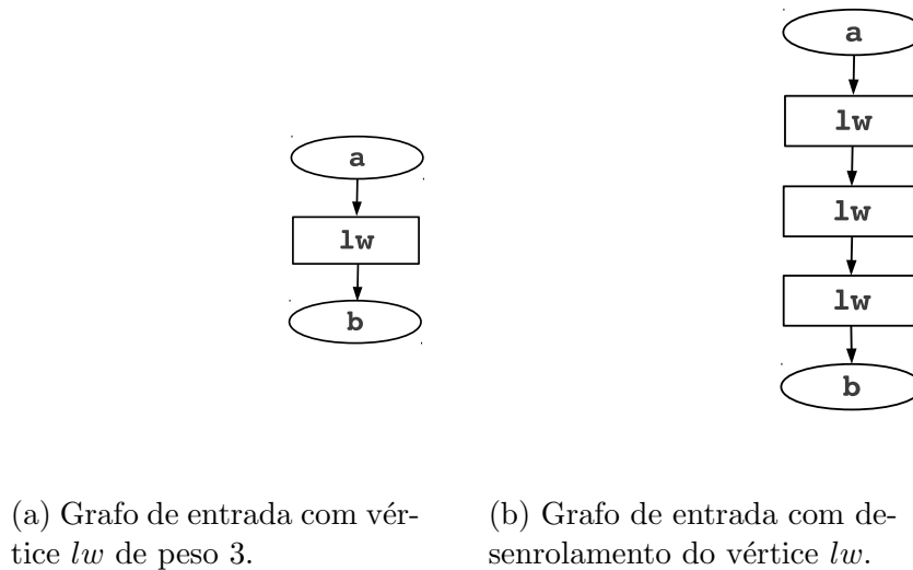
Figura 3.5: Exemplo de desenrolamento do grafo de entrada.
