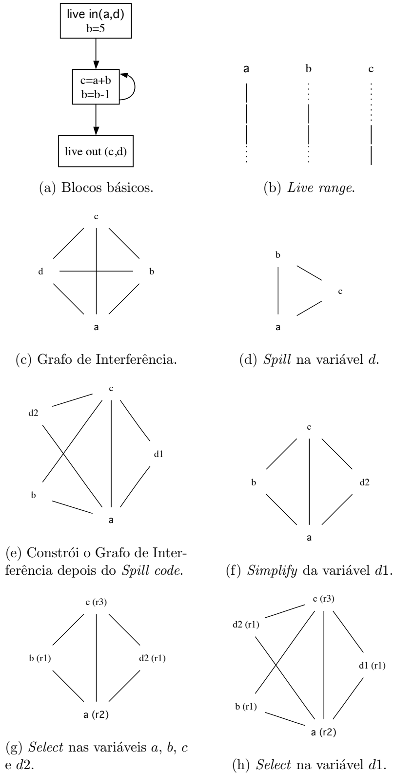
Figura 2.2: Exemplo de alocação de registradores.
