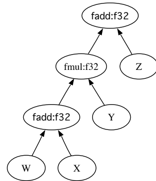
(b) SelectionDAG correspondente.
