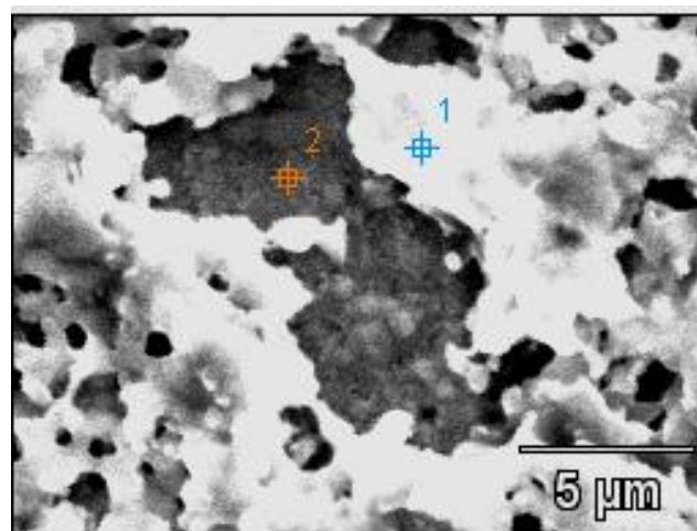
Figura 9 – Região Central indicando os pontos onde foram feitas medidas em EDX no filme de VBA a 1200°C. Ponto 1 (azul) mais distante do substrato cerâmico e Ponto 2 (Laranja) mais próximo ao substrato cerâmico
