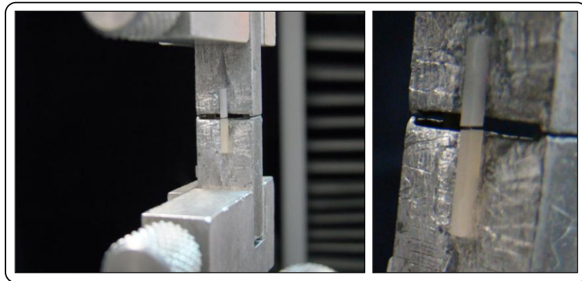
Figura 7 - Teste dos corpos de prova em máquina de ensaios universais
