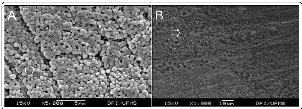
Figura 11 - Superfície das amostras tratadas com 0,5g/10ml VBA a 1400°C. A - Região central mais espessa da amostra com aspecto homogêneo com grãos esféricos (seta) (5000x aumento); B-aspecto esférico dos cristais formados (seta) com interdifusão na matriz (1000x aumento).
