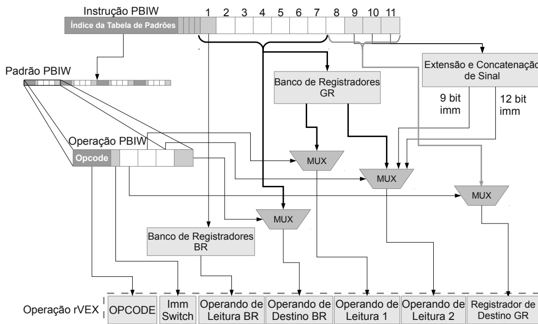
Figura 4.10: Visão geral do decodificador PBIW \rho -VEX versão 1.0.
