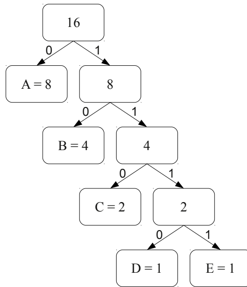
Figura 2.1: Exemplo de árvore de Huffman para a cadeia AAAAAAABBBBCCDE.
