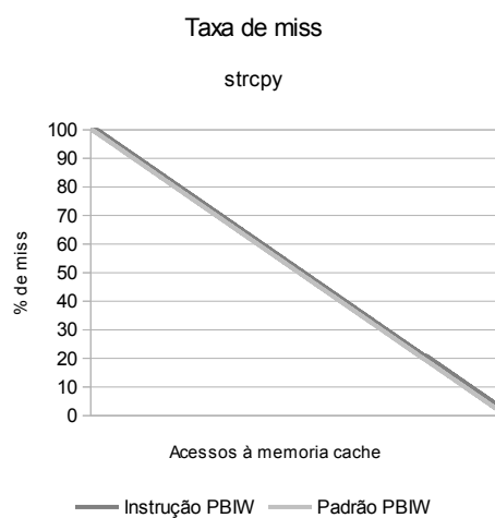
Figura C.2: Taxa de miss para Programas PBIW Versão 2.0
