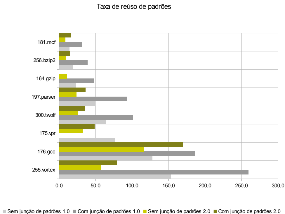
Figura D.2: Taxa de reúso de padrões PBIW para programas SPECINT2000 codificados.
