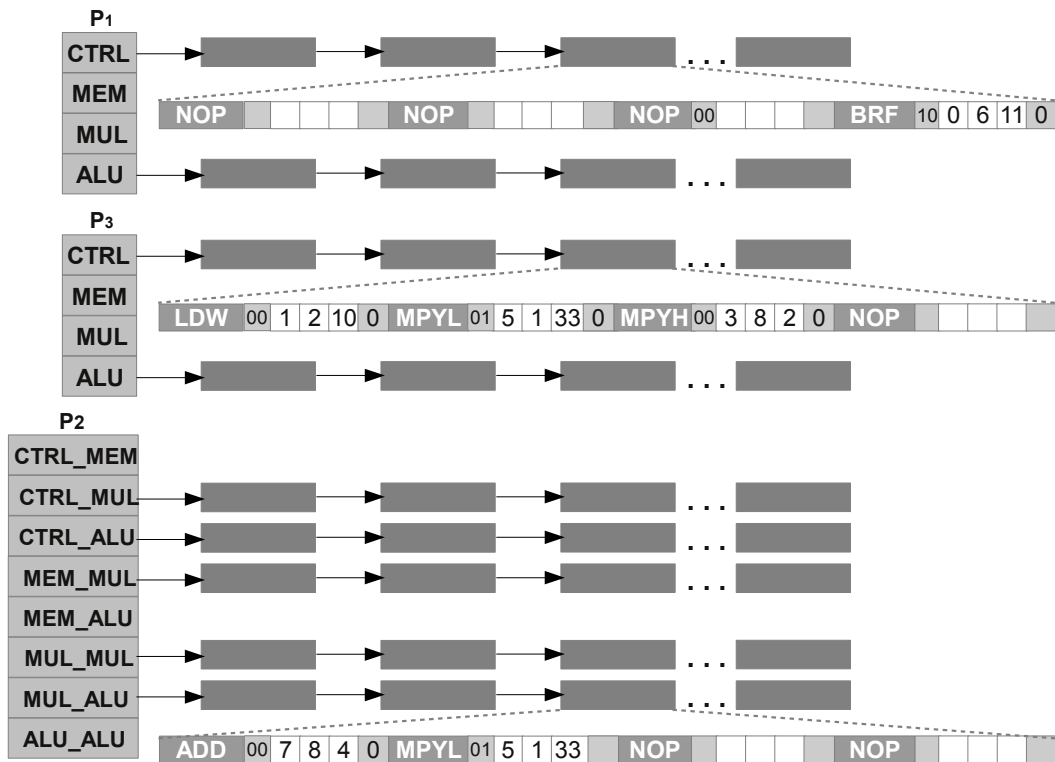
Figura 3.2: Categorias de padrões para o conjunto de instruções VEX.
