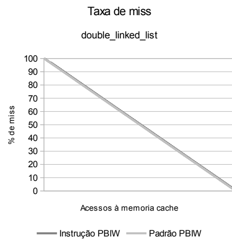
(d) double_linked_list
