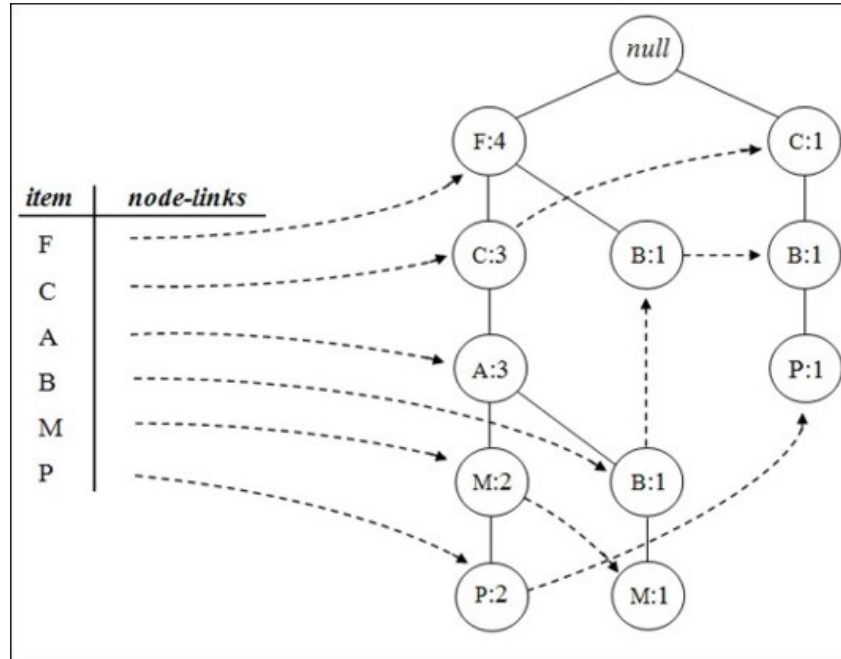
Figura 3.8: FP-Tree construída.
