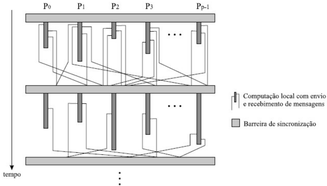
Figura 2.1: Modelo BSP [12]
