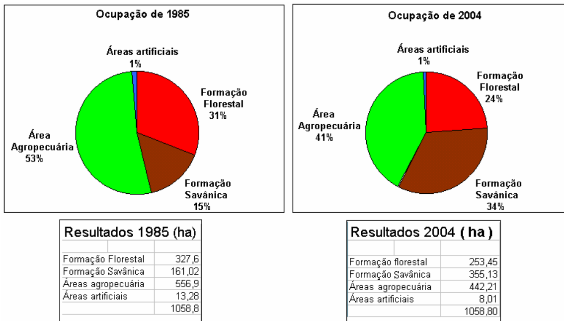
Figura 26: Gráficos da ocupação do solo de 1985 e 2004.
