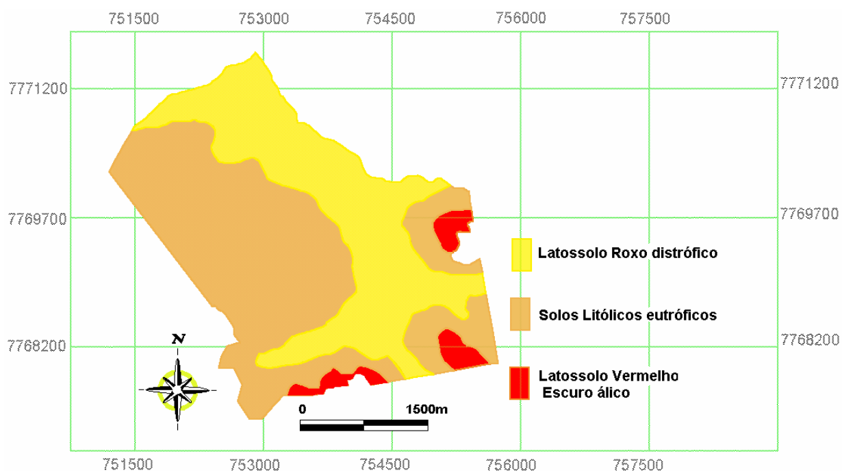
Figura 13: Carta das Associações de Solos de Furnas dos Dionísios. Dados do RADAMBRASIL (BRASIL, 1982) que foram atualizados através da fotointerpretação da banda PAN do LANDSAT ETM+ (LANDSAT, 2002).
