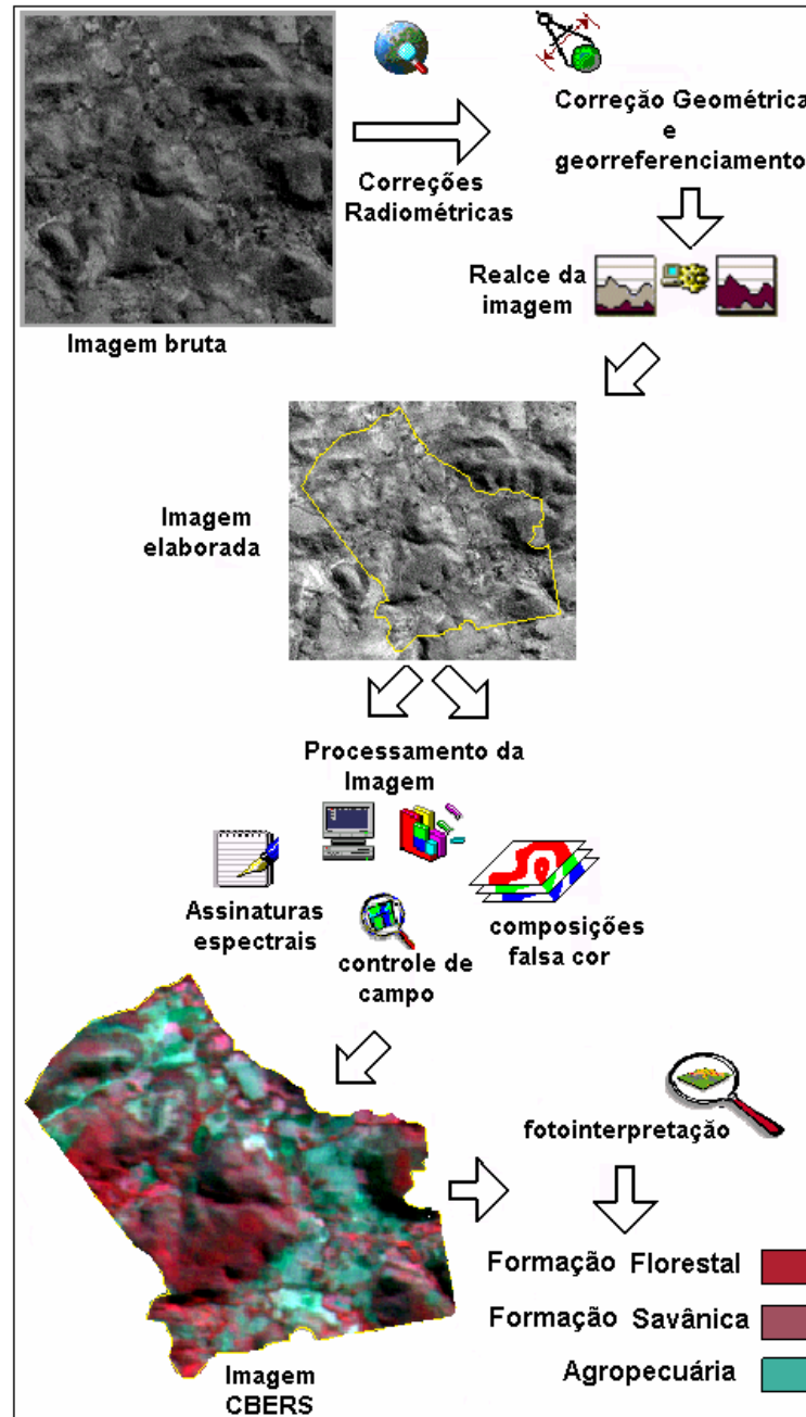
Figura 02: Esquema das etapas de trabalho com imagens de satélite. As imagens foram corrigidas e processadas para possibilitar sua interpretação.
