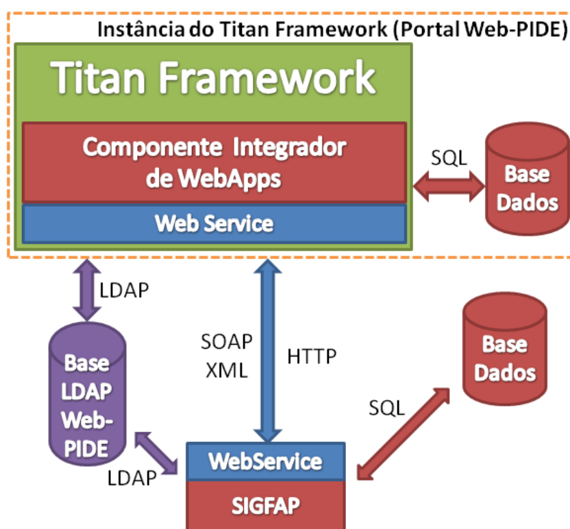
Figura 4.4: Arquitetura projetada para a integração do SIGFAP à plataforma Web-PIDE.
