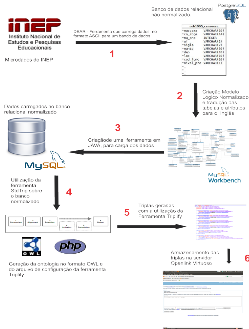
Figura A.9: Etapas para Publicação dos Dados no Padrão Linked Open Data [46].
