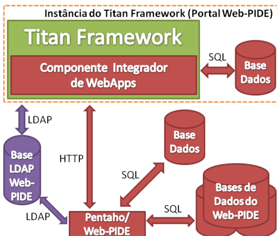
Figura 4.1: Arquitetura projetada para a integração do Pentaho/Web-PIDE ao Portal Web-PIDE.
