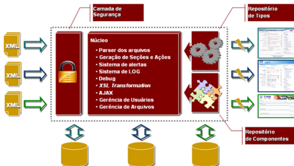
Figura 3.2: Arquitetura do Titan Framework [13].
