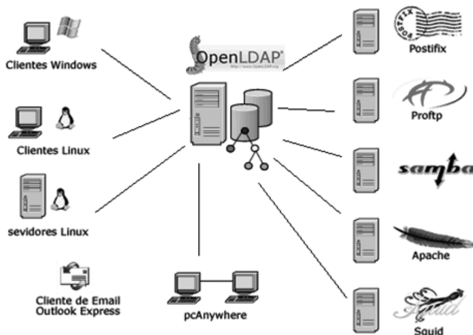
Figura 3.3: Utilização do LDAP como base para diversos serviços na rede [2].
