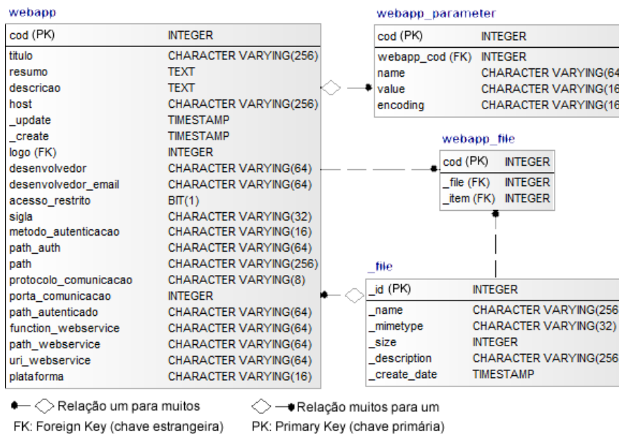
Figura 3.8: Modelagem do banco de dados do AIA.
