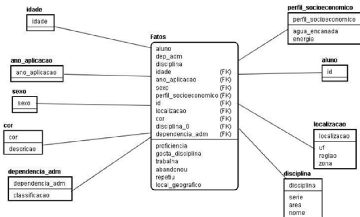
Figura A.6: Cubo SAEB gerado utilizando JUDE/Java [40].
