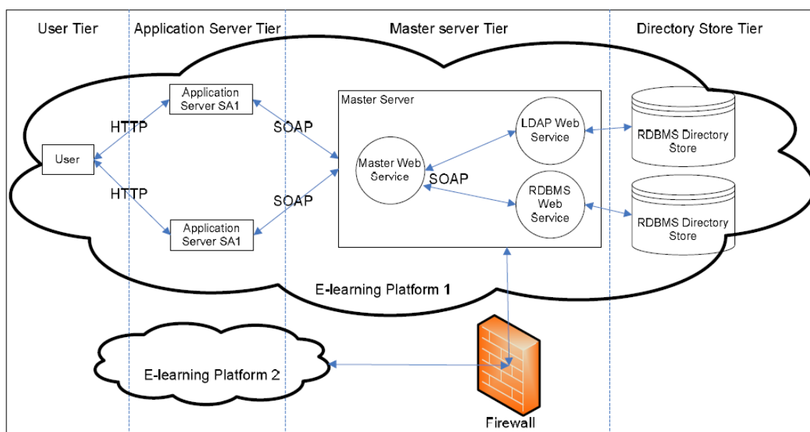
Figura 5.2: Arquitetura do WSAS com a integração de plataformas de EAD [1].
