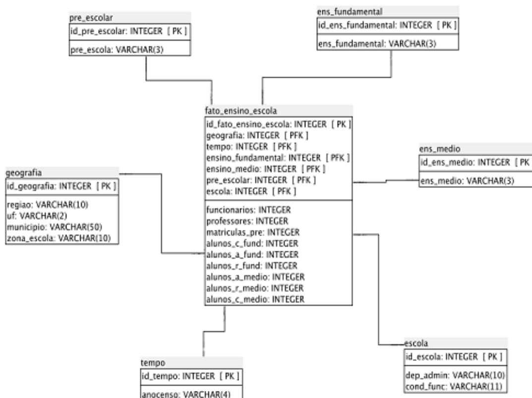
Figura A.7: Cubo CEB gerado utilizando JUDE/Java [47].
