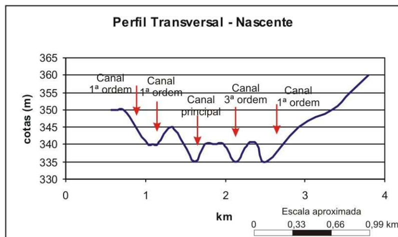
Figura 12: Perfil Transversal da nascente da sub-bacia Córrego São Roberto.
