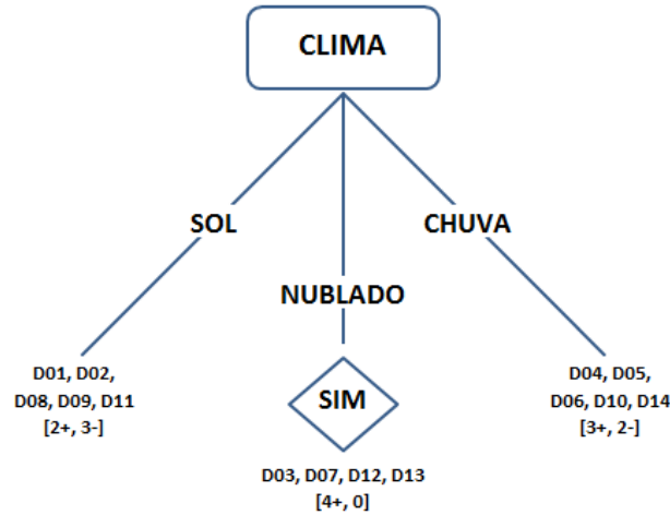
Figura 2.2: Árvore iniciada com o atributo de maior ganho de informação
