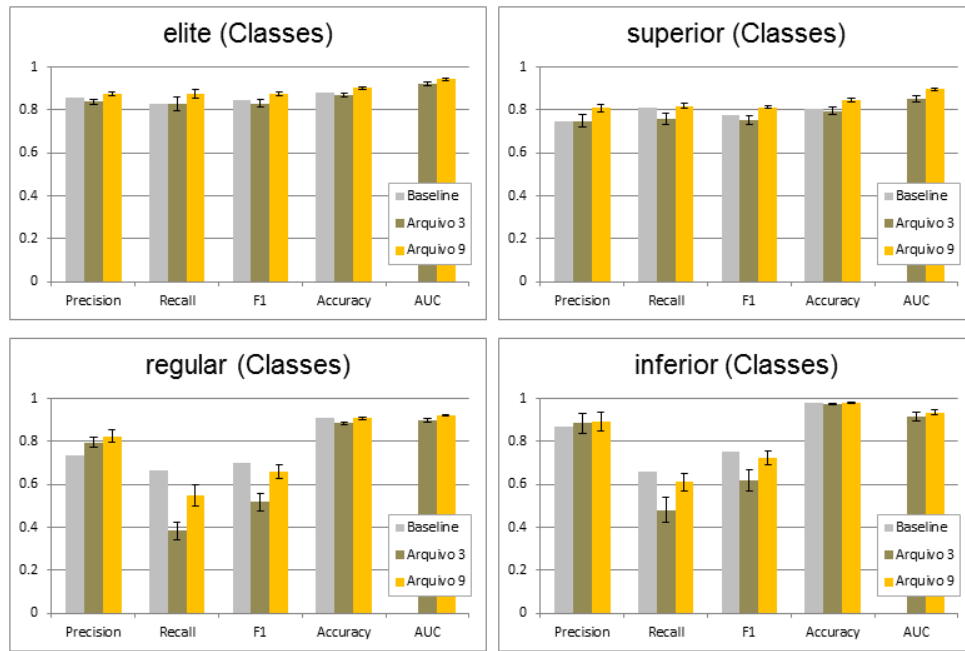
Figura 3.10: Gráficos comparativos para os conjuntos de dados de Classes da Rodada 1 (Arquivo 3) e da Rodada 4 (Arquivo 9). No topo das barras estão representados o desvio-padrão ( Standard Deviation )
