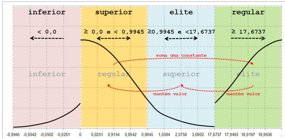
Figura 3.26: Conversor para EscoreR
