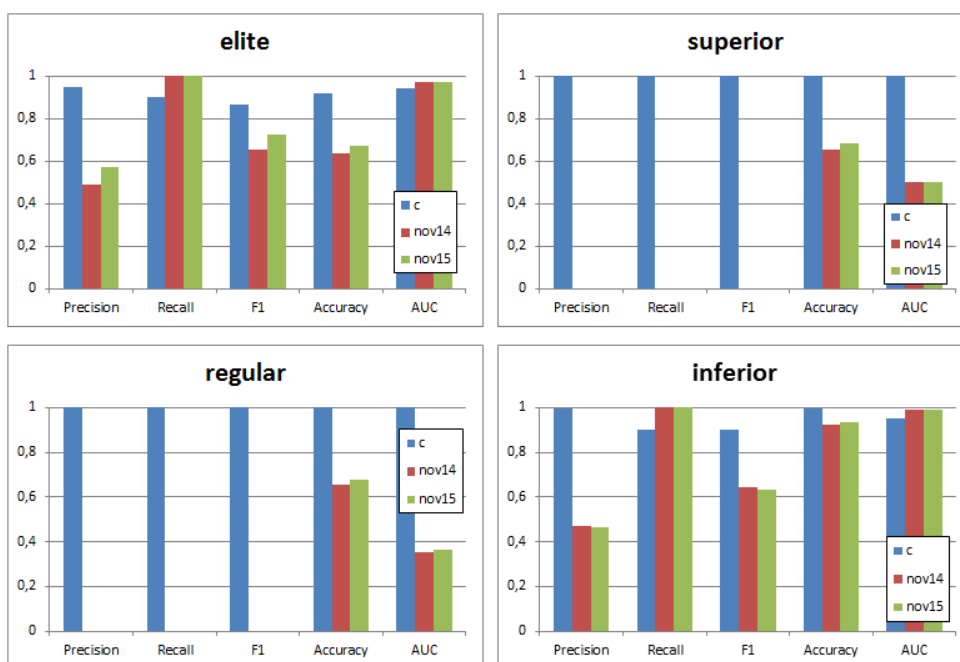
Figura 3.30: Comparativo do reaproveitamento do classificador nas avaliações de Novembro 2014 e Novembro 2015
