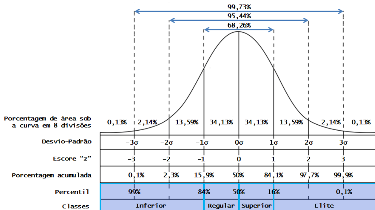
Figura 3.21: Curva normal e classes
