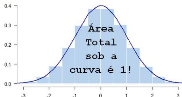
Figura 3.19: Propriedades da Normal Padrão
