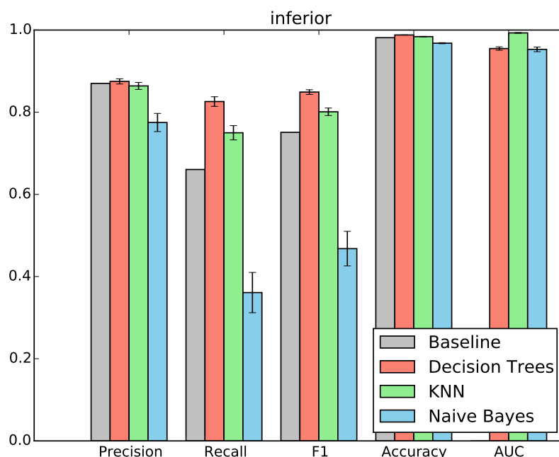
Figura 3.14: Comparativo de indutores para classe inferior . No topo das barras estão representados o erro padrão ( Standard Error )
