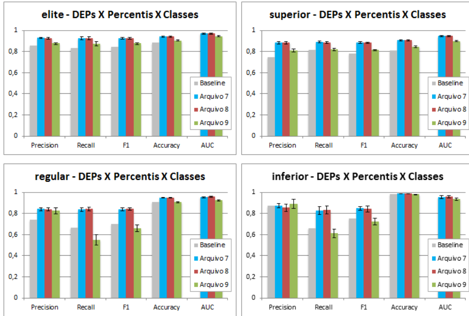
Figura 3.7: Gráficos comparativos para a Rodada 4. No topo das barras estão representados o desvio-padrão ( Standard Deviation )
