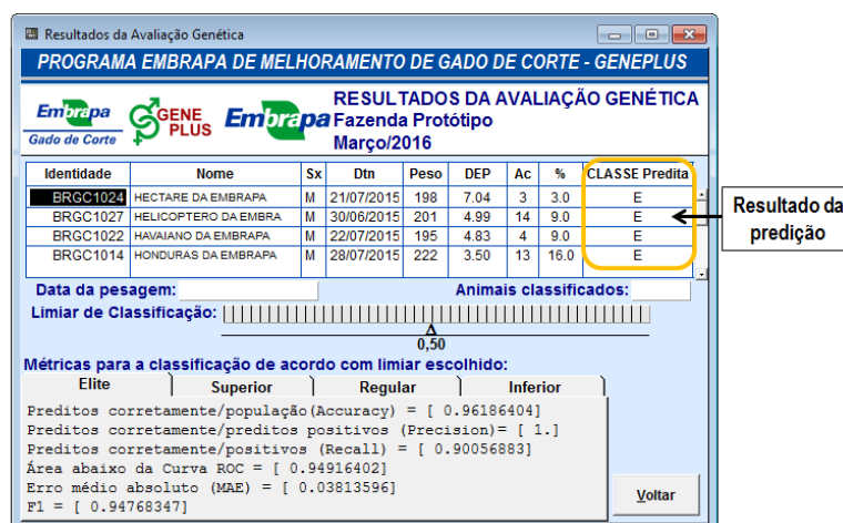
Figura 4.4: Tela Final - Resultados da classificação via SICADEB
