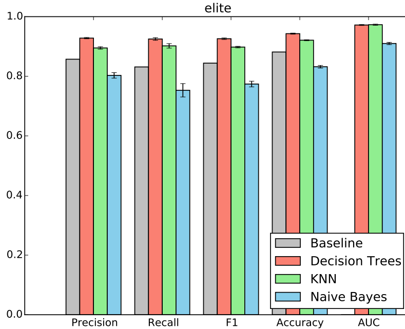
Figura 3.11: Comparativo de indutores para Classe elite . No topo das barras estão representados o erro padrão ( Standard Error )
