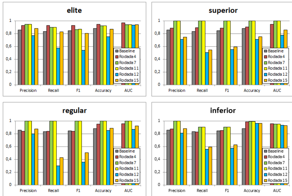
Figura 3.31: Resultados para o uso do PDaju como atributo: baseline = resultados baseados na predição da Classe da DEP_{\text{PaiMãe}} ; Rodada 4 = resultados antes de incluir os escores; Rodada 7 = resultados após incluir os escores; Rodada 11 = resultados com escores e sem PDaju; Rodada 12 = resultados sem escores e sem PDaju; e Rodada 15 = resultados sem escores e com PDaju
