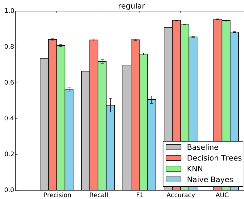
Figura 3.13: Comparativo de indutores para classe regular . No topo das barras estão representados o erro padrão ( Standard Error )
