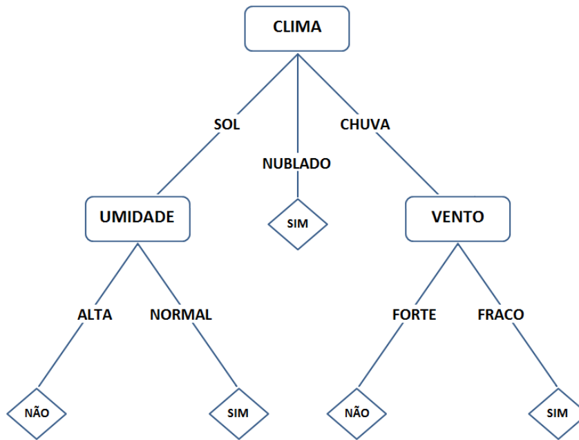
Figura 2.3: Árvore de decisão construída segundo o ganho de informação
