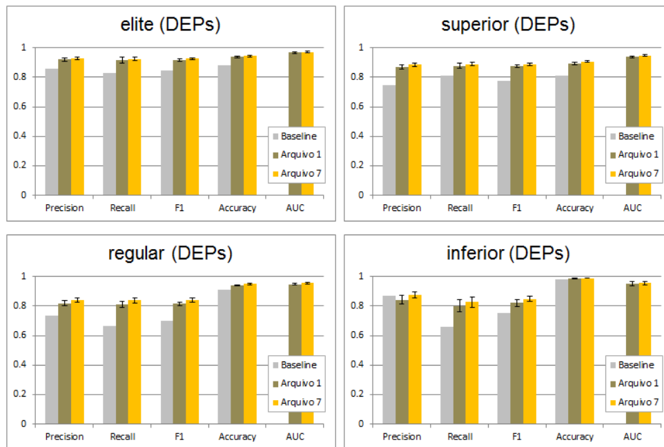
Figura 3.8: Gráficos comparativos para os conjuntos de dados de DEPs da Rodada 1 (Arquivo 1) e da Rodada 4 (Arquivo 7). No topo das barras estão representados o desvio-padrão ( Standard Deviation )
