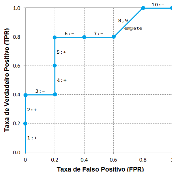
Figura 2.5: Curva ROC para o exemplo
