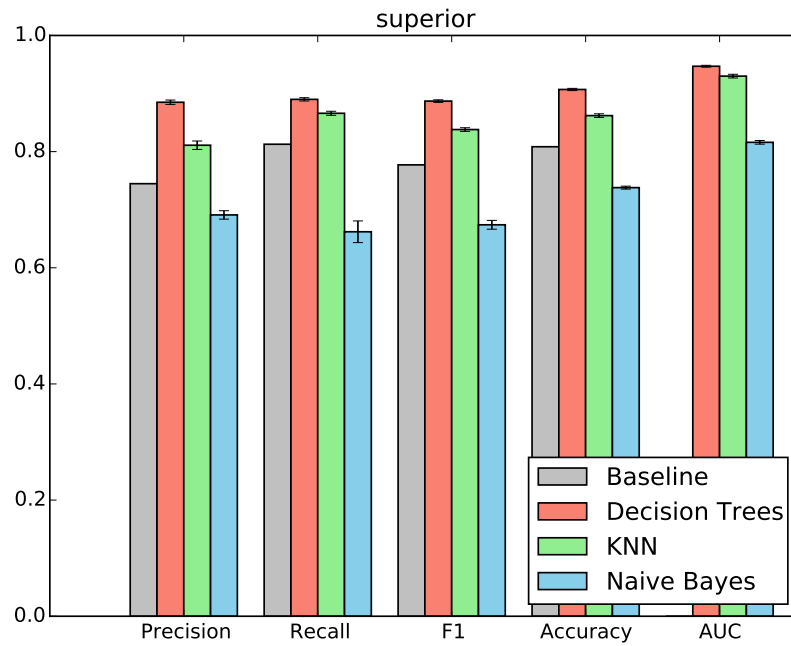
Figura 3.12: Comparativo de indutores para classe superior . No topo das barras estão representados o erro padrão ( Standard Error )
