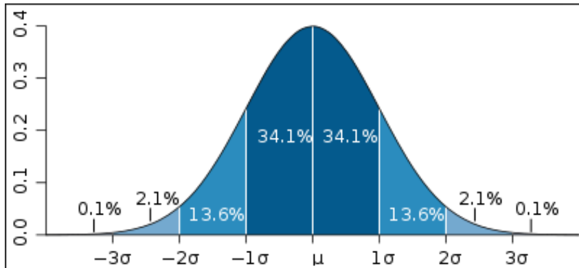
Figura 3.16: Curva normal e desvio-padrão Fonte: Wikipedia 4
