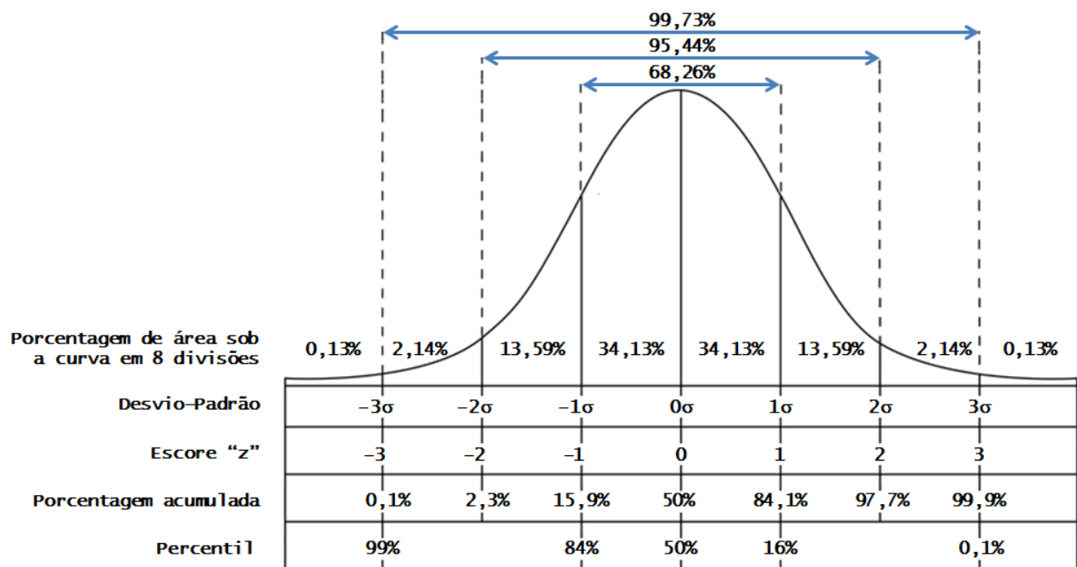
Figura 3.20: Curva normal e intervalos
