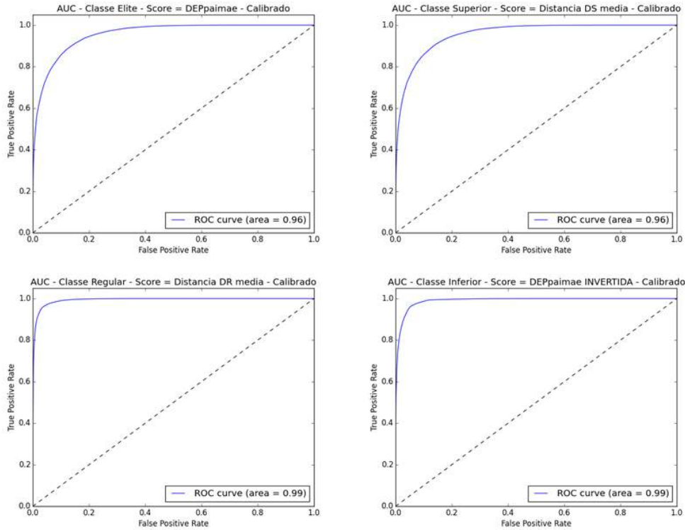
Figura 3.27: Gráficos ROC para as classes elite, superior, regular e inferior utilizando escores
