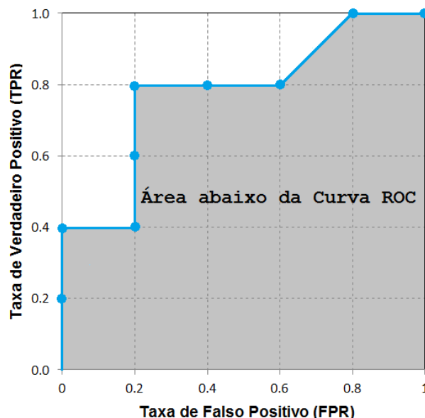
Figura 2.6: Área abaixo da curva ROC - AUC para o exemplo
