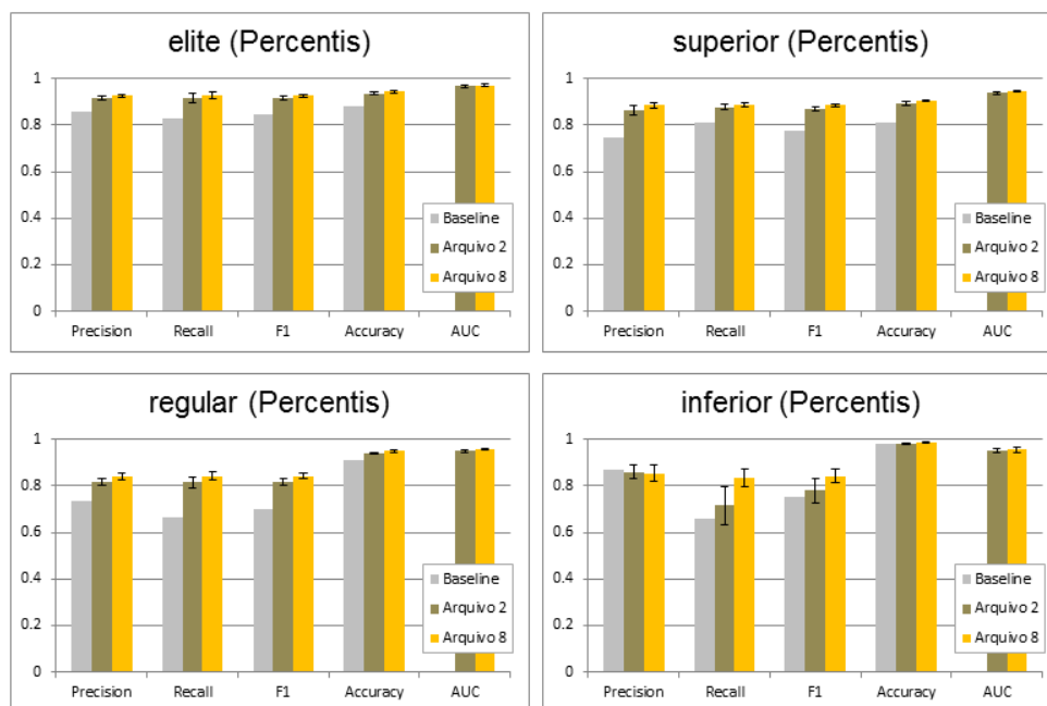
Figura 3.9: Gráficos comparativos para os conjuntos de dados de Percentis da Rodada 1 (Arquivo 2) e da Rodada 4 (Arquivo 8). No topo das barras estão representados o desvio-padrão ( Standard Deviation )
