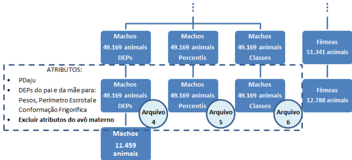
Figura 3.5: Refinamento dos atributos: Eliminação dos referentes ao avô materno
