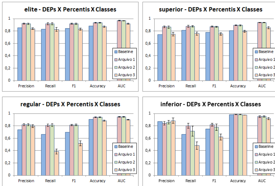
Figura 3.4: Gráficos comparativos para a Rodada 1. No topo das barras estão representados o desvio-padrão ( Standard Deviation )
