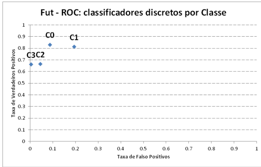
Figura 3.1: Gráfico ROC para o desempenho Classe_{PaiMãe}
