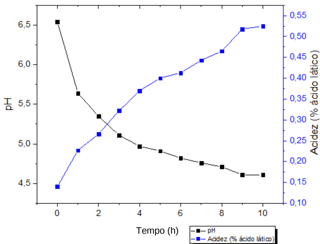
Figura 7 - Curva de fermentação, EHB com adição de 12% de sacarose.
