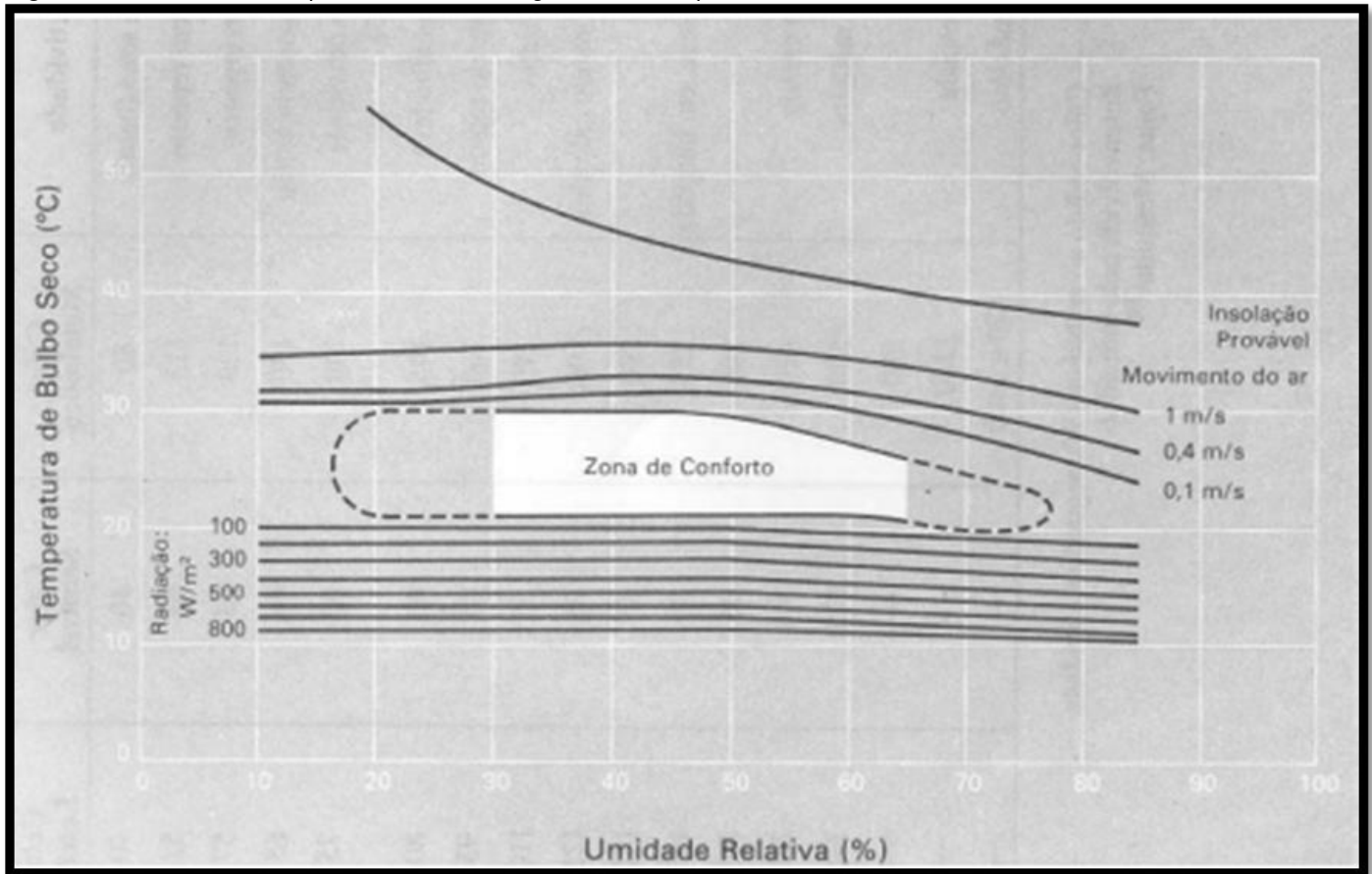
Figura 8: Carta Bioclimática para habitantes de regiões de clima quente.
