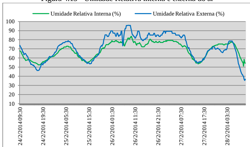
Figura 4.13 - Umidade Relativa interna e externa do ar
