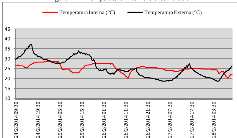
Figura 4.7 - Temperatura interna e externa do ar
