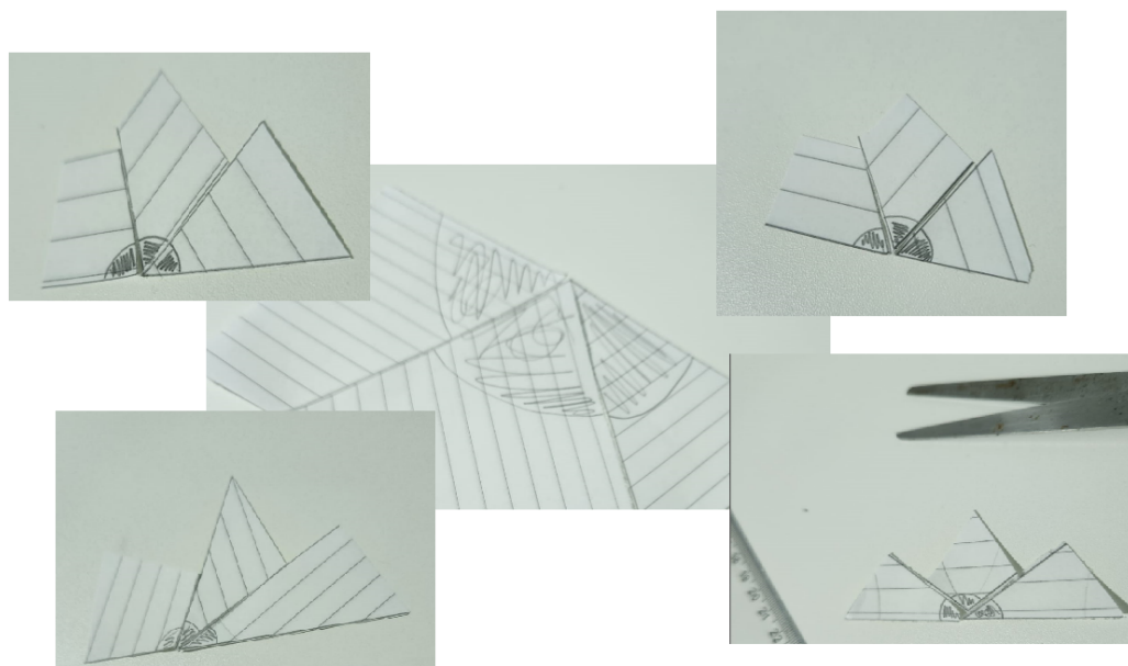
Figura 25 – Soma dos Ângulos Internos de um Triângulo na Prática
