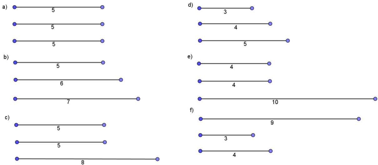
Figura 4 – Medidas dos Lados
