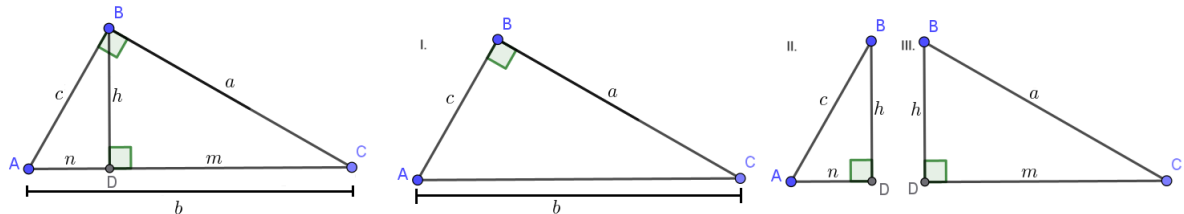
Figura 22 – Triângulos Semelhantes a partir de um Triângulo Retângulo
