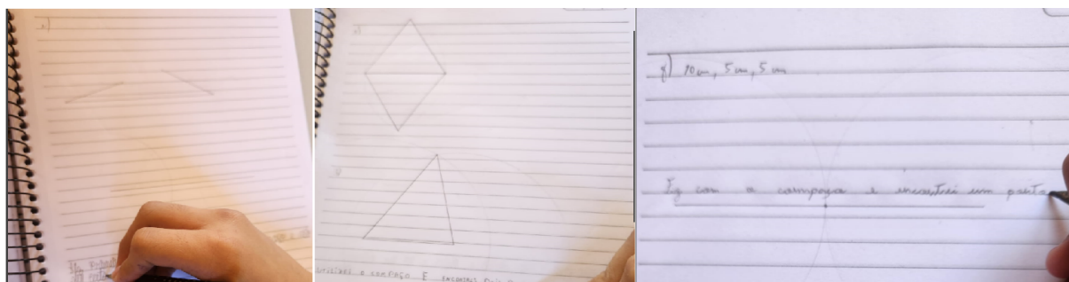
Figura 24 – Construções com Compasso e Formação de Triângulos quando Possível
