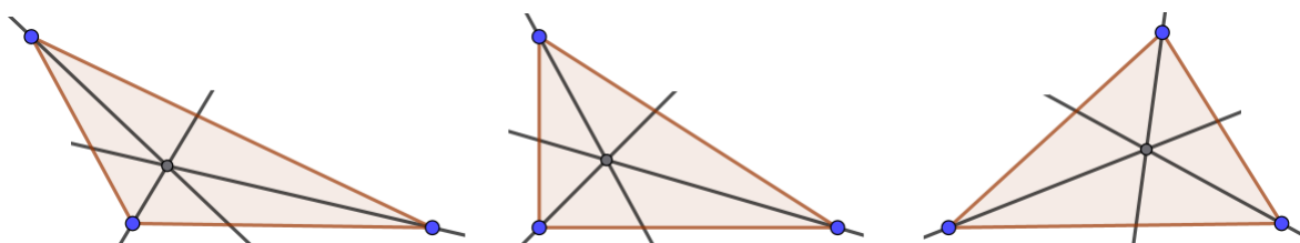
Figura 16 – Incentros
