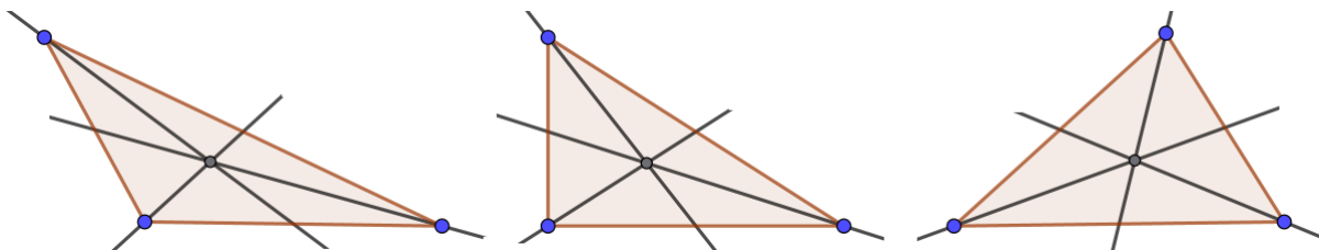
Figura 15 – Baricentros
