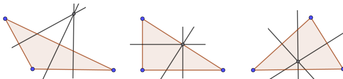
Figura 18 – Circuncentros
