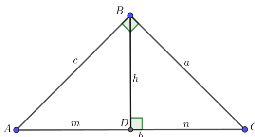
Figura 31 – Triângulo ABC
