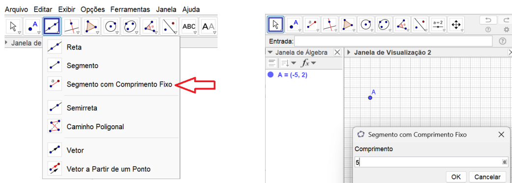
Figura 6 – Segmento com Comprimento Fixo
