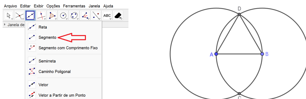
Figura 10 – Segmento e Triângulos Formados
