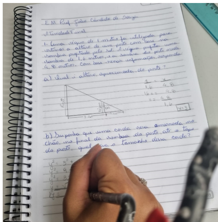
Figura 33 – Resoluções
