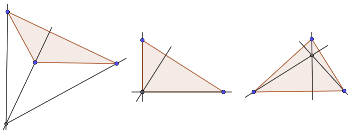
Figura 17 – Ortocentros
