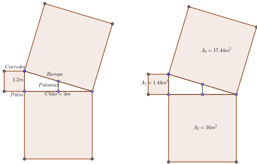
Figura 21 – Teorema de Pitágoras
