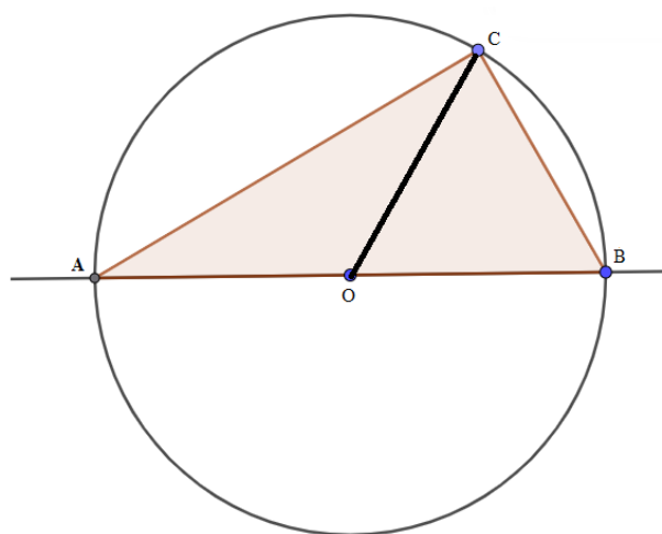
Figura 64 – Divisão mereológica no triângulo ABC
