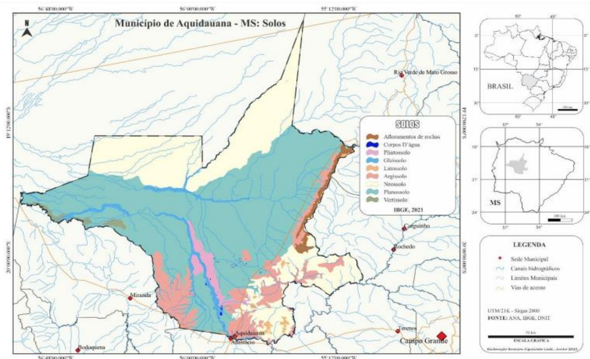
FIGURA 4: MUNICÍPIO DE AQUIDAUANA-MS: SOLOS
