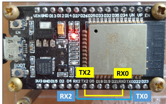
Figura 5. Conexão física entre interfaces de comunicação Serial. Fonte: Autoria própria.
