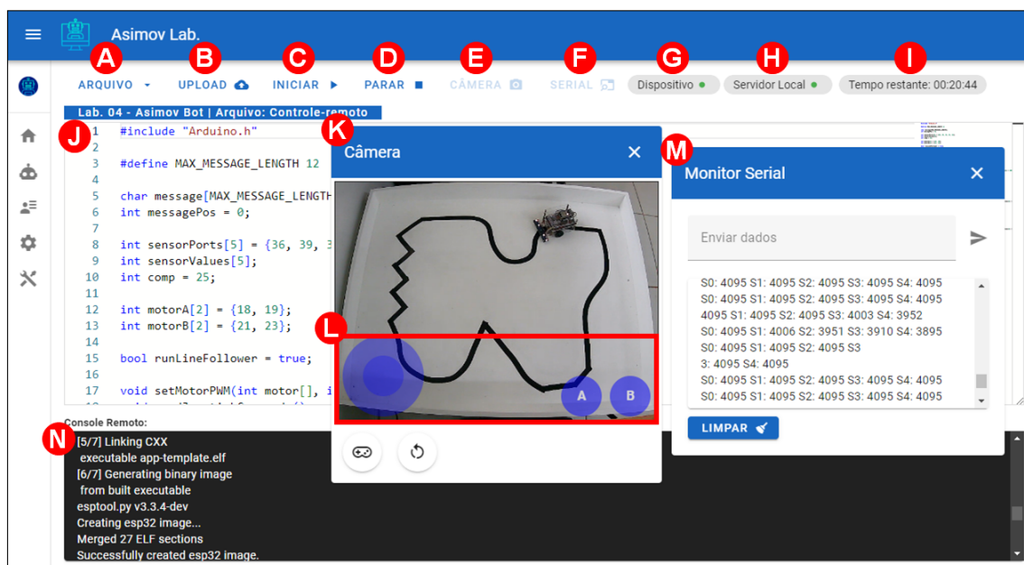
Figura 8. Interface gráfica do experimento. Fonte: Autoria própria.
