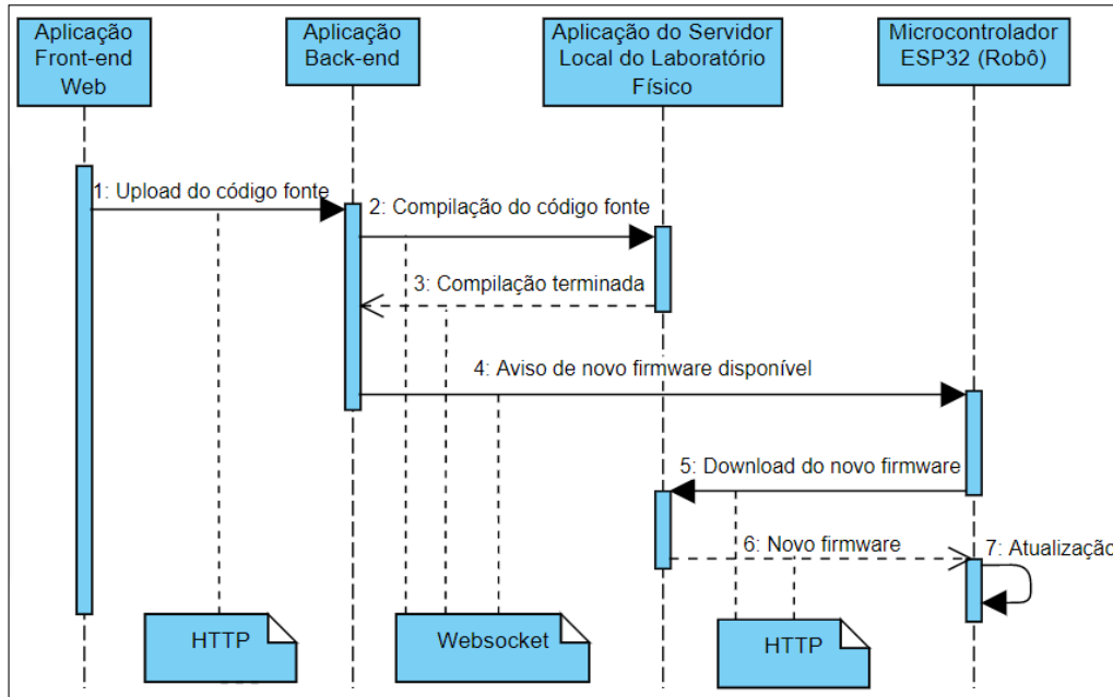
Figura 3. Diagrama de sequência. Fonte: Autoria própria.
