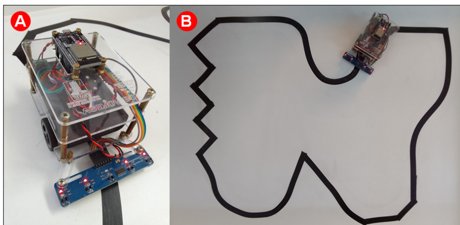
Figura 12. Dispositivo do experimento 3. A - Robô seguidor de linha com array de sensores reflexivos infravermelho, par de motores N20 75 RPM 3v, ponte H dupla L298N e powerbank de 5v e 10000 mAH. B - Pista para o robô seguidor de linha. Fonte: Autoria própria.
