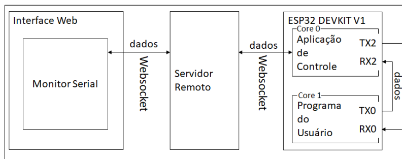
Figura 6. Os dados trafegam pela internet através de websockets e são retransmitidos pelos pares de portas RX/TX da placa ESP32 DEVKIT V1 pela aplicação de controle. Fonte: Autoria própria.
