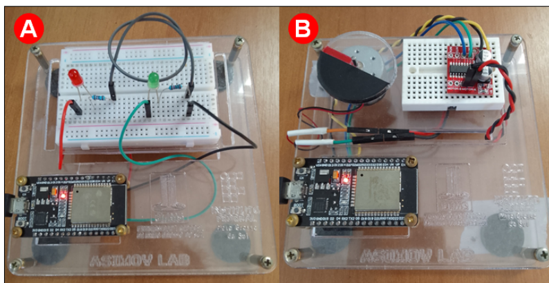
Figura 11. Dispositivos dos experimentos 1 e 2. A - circuito simples com dois leds. B - circuito com um motor DC e modulo de ponte H dupla L298N. Fonte: Autoria própria.
