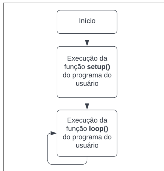
Figura 10. Fluxograma da tarefa secundária da aplicação de controle. Fluxo executado pelo segundo núcleo do processador do ESP32. Fonte: Autoria própria.
