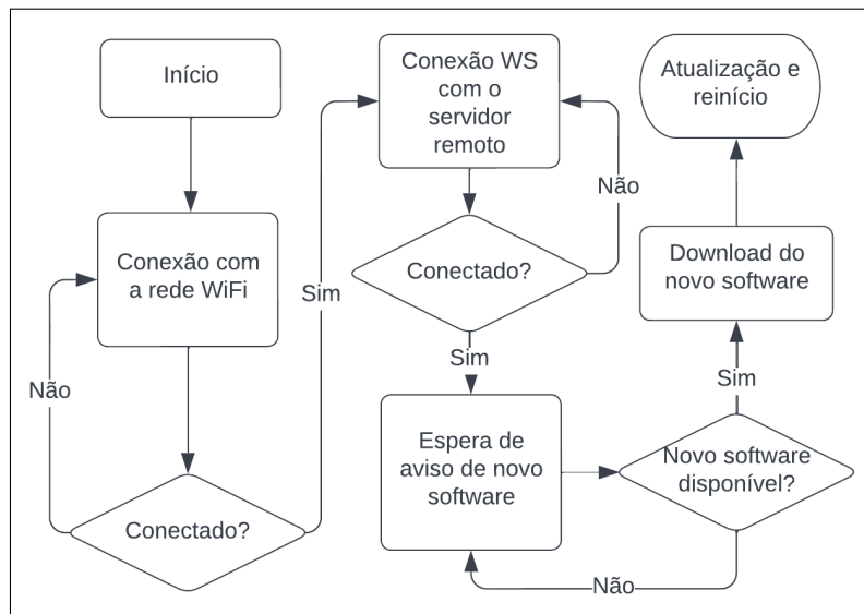
Figura 9. Fluxograma da tarefa principal da aplicação de controle. Fluxo executado pelo primeiro núcleo do processador do ESP32. Fonte: Autoria própria.
