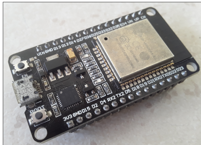
Figura 2. Placa de desenvolvimento ESP32 DEVKIT V1. Fonte: Autoria própria.
