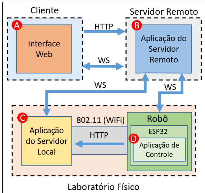
Figura 1. Esquema da arquitetura do sistema desenvolvido. Fonte: Autoria própria.
