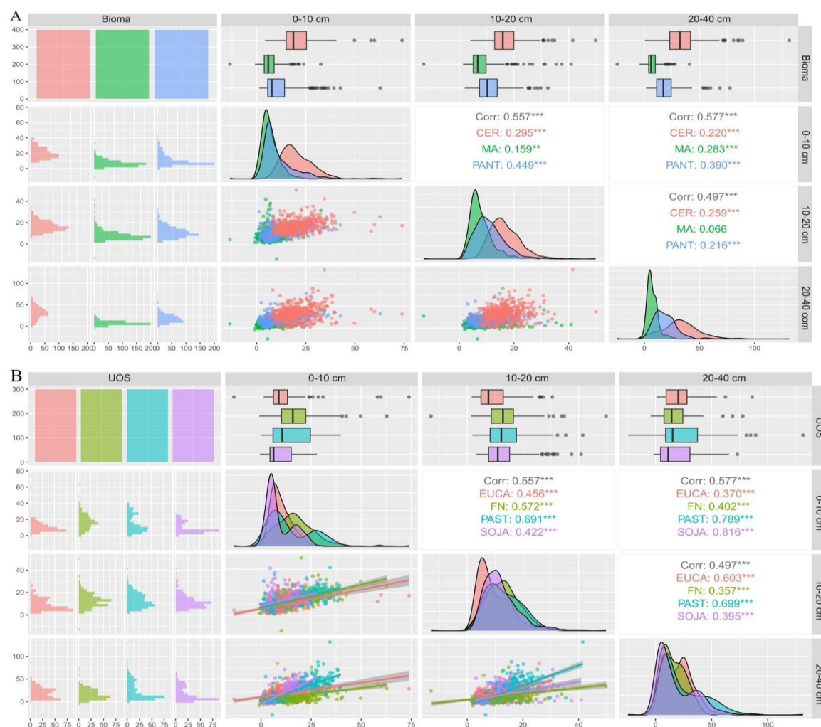
Figura 3. Análise de correlação de Pearson para a variável estoque de carbono avaliada em diferentes usos e ocupação do solo nos biomas Cerrado (CER), Mata Atlântica (MA) e Pantanal (PANT) de Mato Grosso do Sul.
