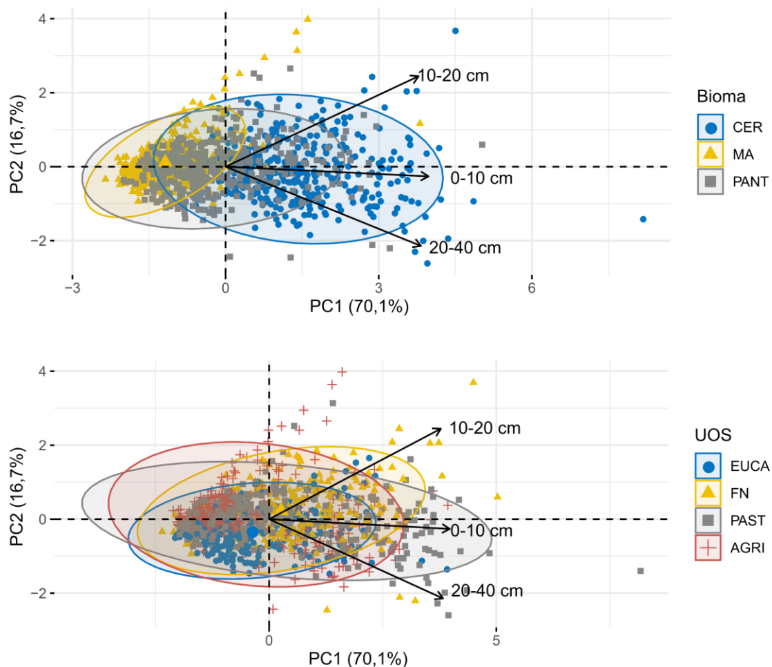
Figura 2. Análise de componentes para a variável estoque de carbono avaliada em diferentes usos e ocupação do solo nos biomas de Mato Grosso do Sul.
