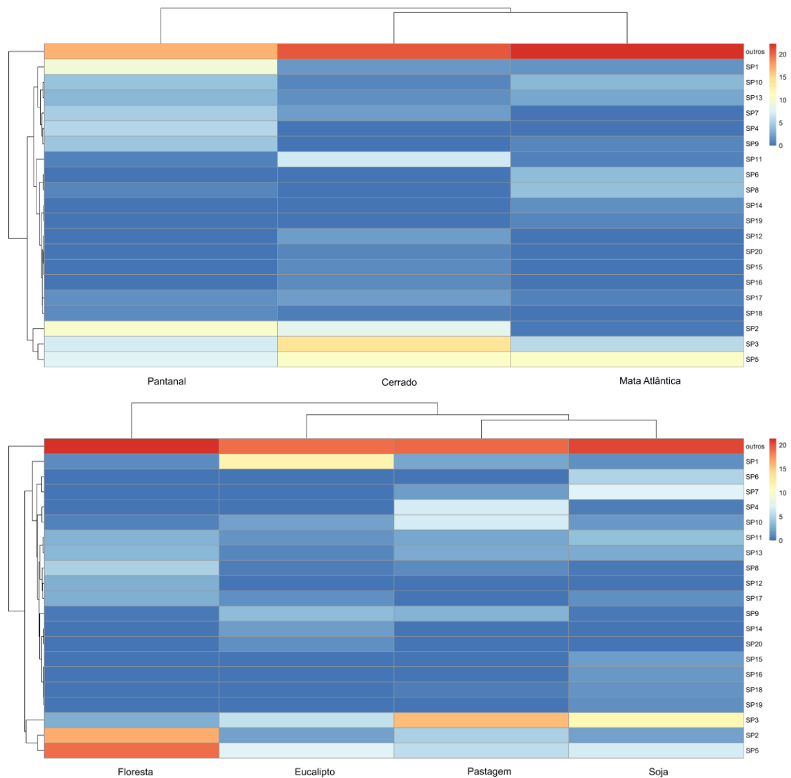
Figura 4. Heatmap para relação entre s fungos nos biomas (A) e usos (B) das amostras de solo avaliadas.
