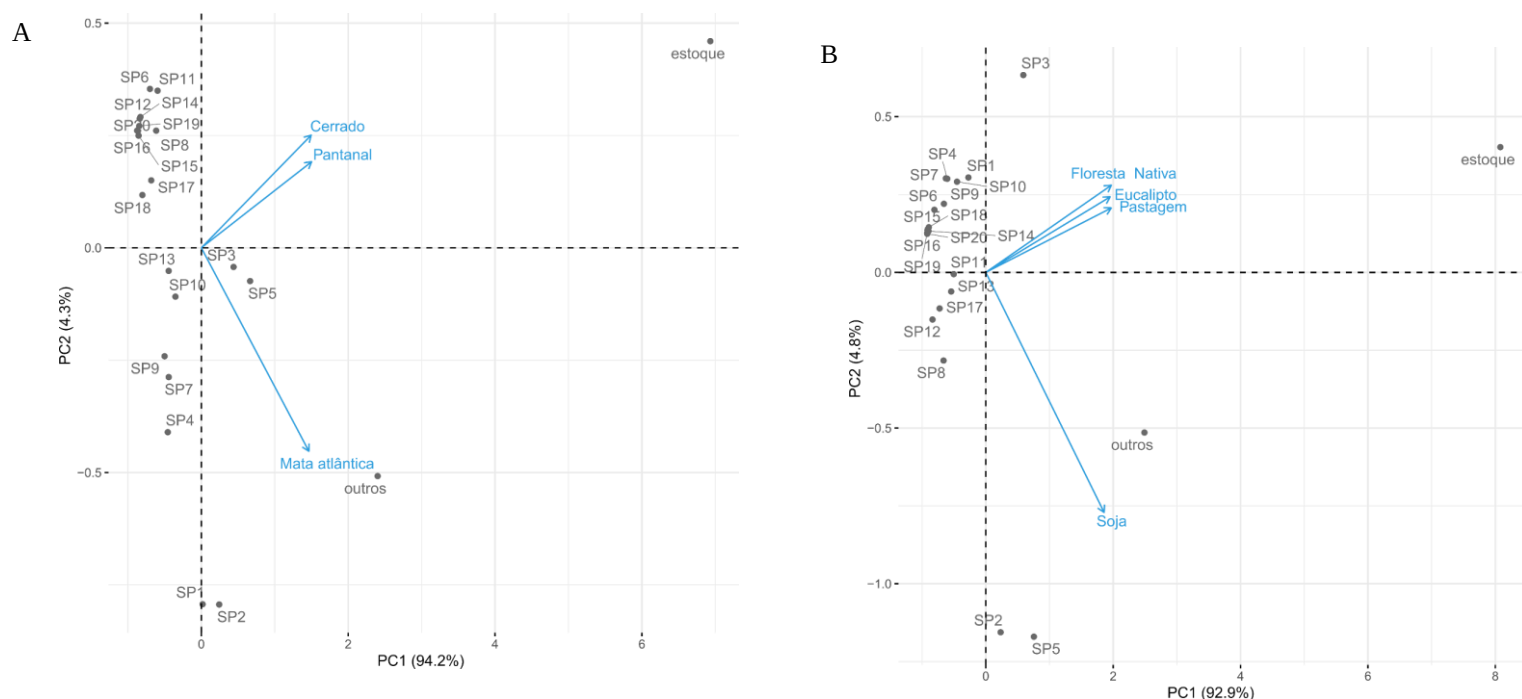
Figura 2. Análise de componentes principais para os fungos presente nas amostras e o estoque de carbono para os biomas Cerrado, Pantanal e Mata atlântica (A) e nos usos eucalipto, agricultura (soja), pastagem e floresta nativa (B).
