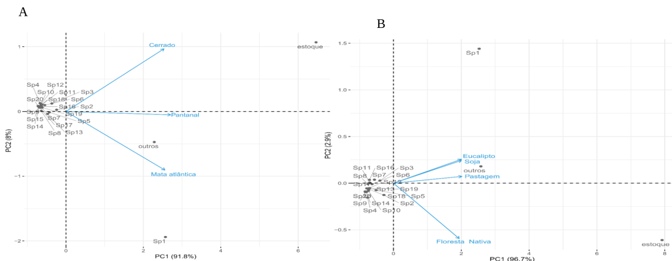
Figura 1. Análise de componentes principais para as bactérias presente nas amostras e o estoque de carbono para os biomas Cerrado, Pantanal e Mata atlântica (A) e nos usos eucalipto, agricultura (soja), pastagem e floresta nativa (B).
