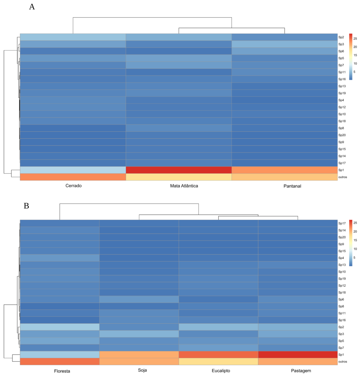
Figura 3. Heatmap para relação entre as bactérias nos biomas (A) e usos (B) das amostras de solo avaliadas
