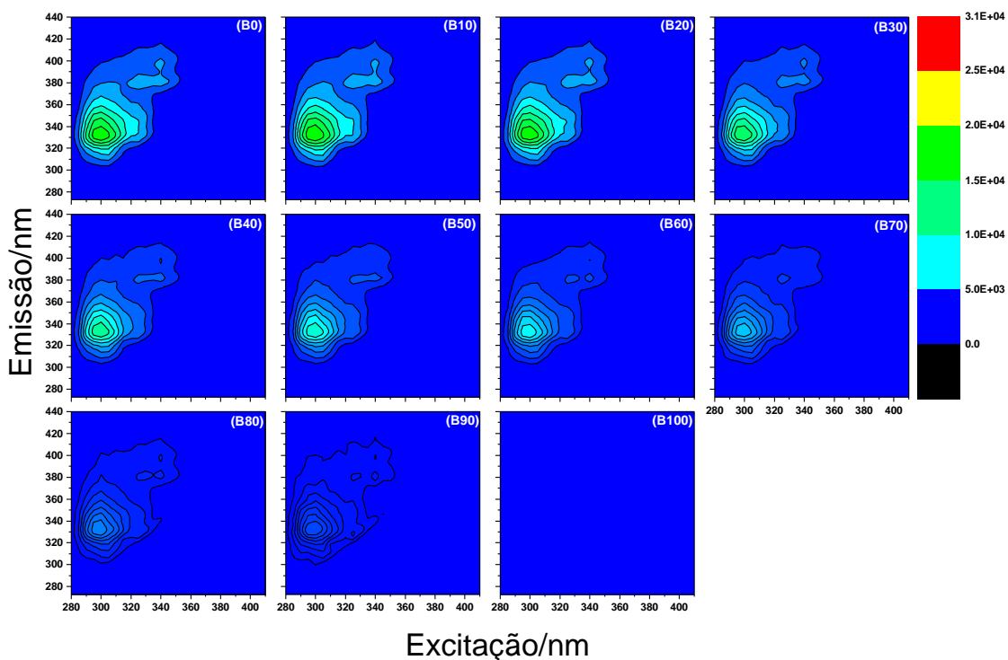
Figura 29 - MEEp(D) das blendas de diesel biodiesel diluídas em solução de EGTW80 obtidas para a polarização HH. A escala de cores corresponde aos valores de intensidade de fluorescência.
