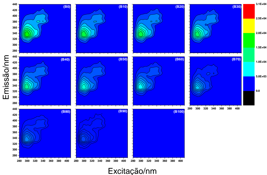
Figura 28. MEEp(D) das blendas de diesel biodiesel diluídas em solução de EGTW80 obtidas para a polarização HV. A escala de cores corresponde aos valores de intensidade de fluorescência.
