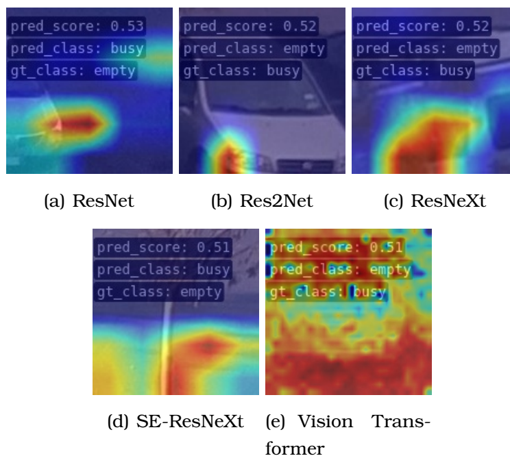
Figura 4.4: Mapa de ativação das imagens erradas.
