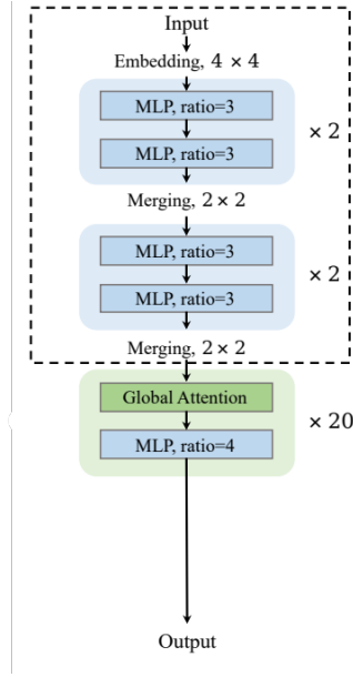
Figura 3.10: Imagem ilustrativa do HiViT.
