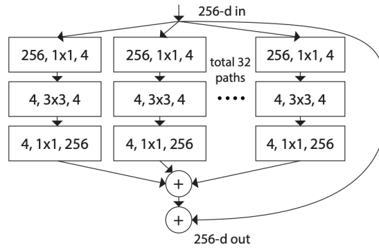
Figura 3.5: Bloco da ResNeXt com cardinalidade 32.
