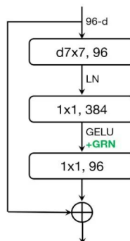
ConvNeXt V2 Block
