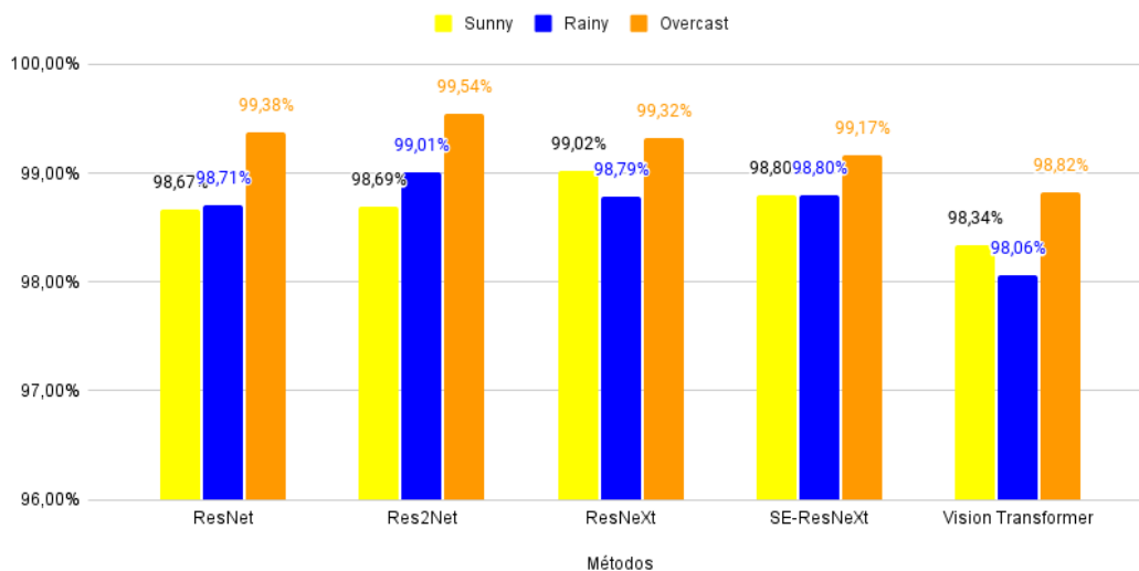
Figura 4.1: Precisão dos modelos de acordo com a condição climática.
