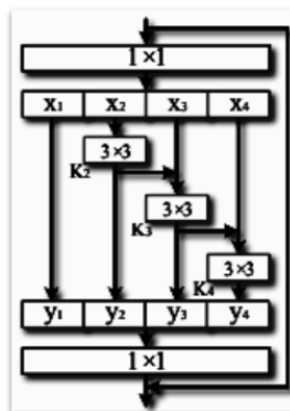
Figura 3.7: Imagem ilustrativa da Res2Net.
