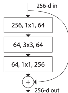
Figura 3.4: Bloco da ResNet.
