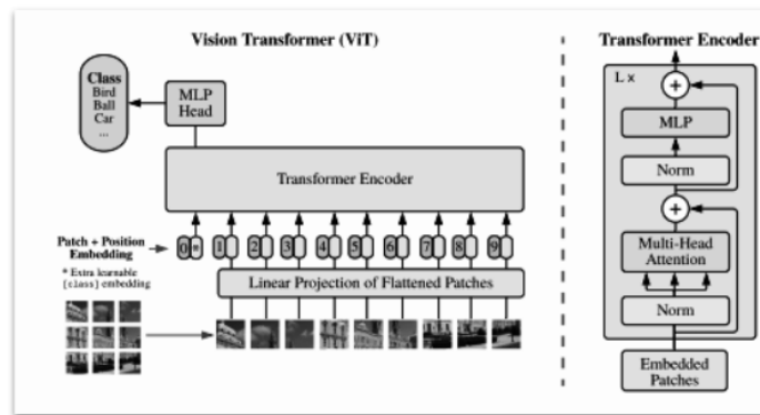
Figura 3.9: Imagem ilustrativa do Vision Transformer .
