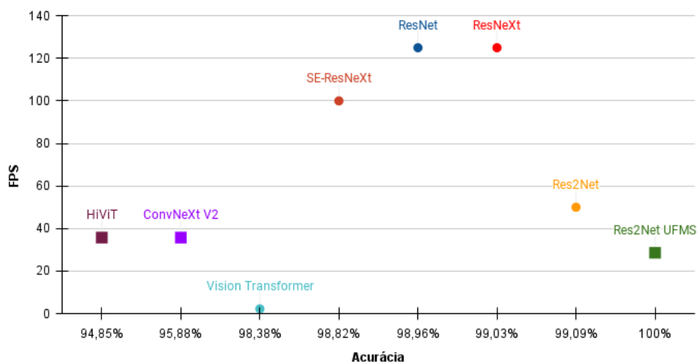
Figura 4.7: FPS x Taxa de Acerto.
