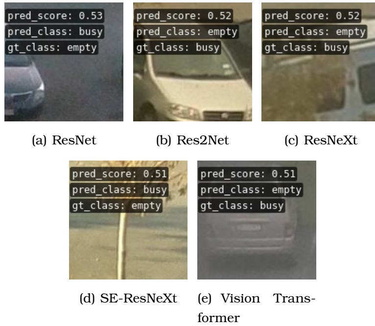
Figura 4.3: Exemplos de erros dos modelos.
