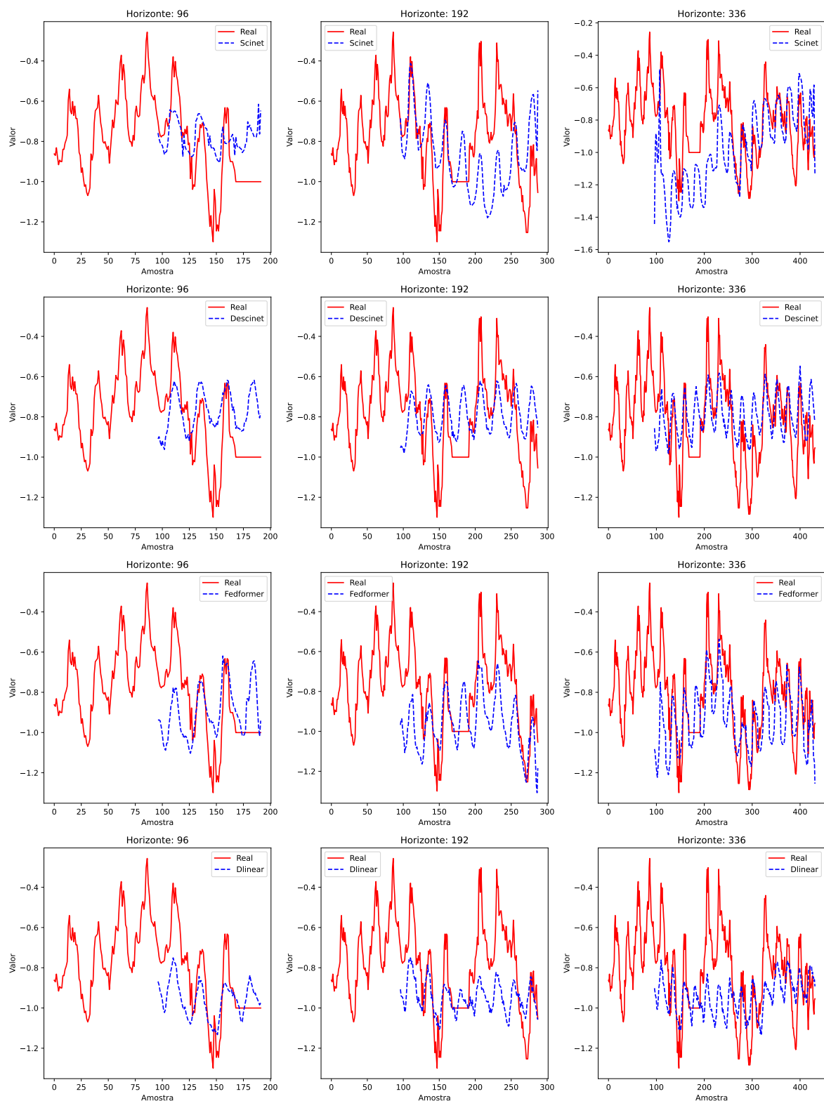
Figura 5.5: Comparativo de previsão para os horizontes de 96, 192 e 336 entre os algoritmos DESCINet, SCINet, FEDformer e DLinear no conjunto de dados univariado ETTh1.
