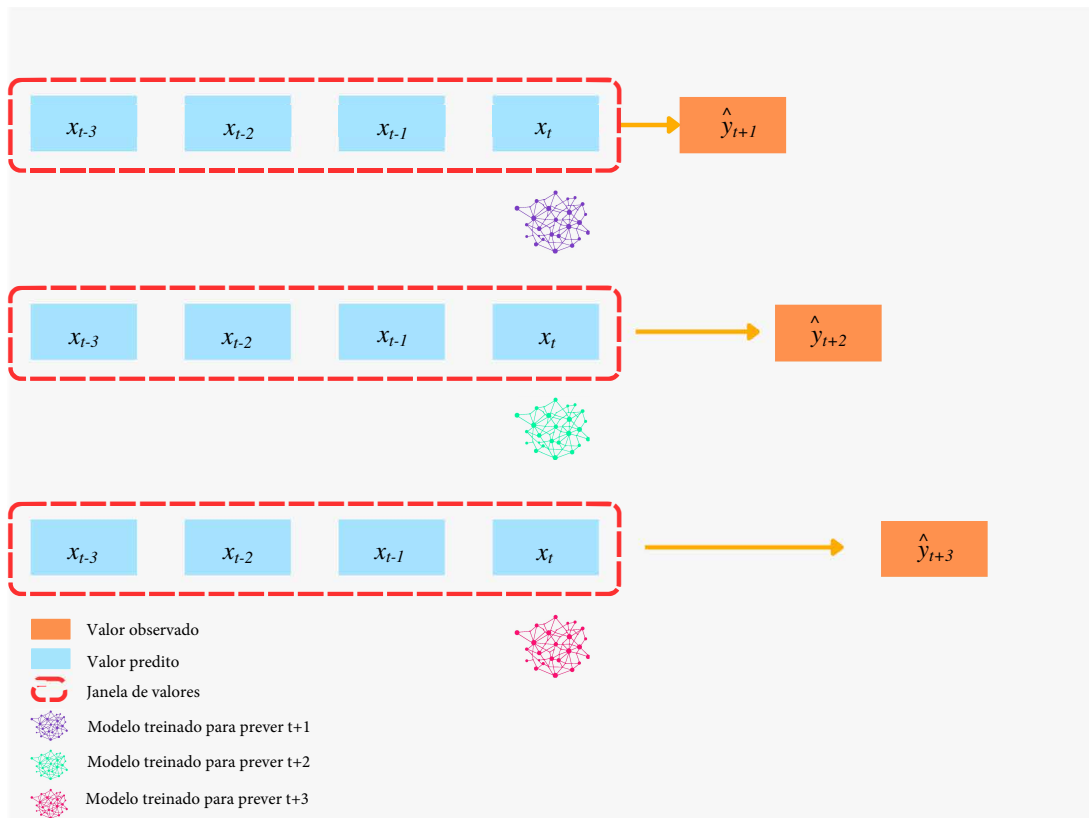
Figura 2.12: Ilustração do funcionamento do método DMS
