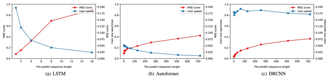
Figura 3.1: Desempenho do modelo no ETTm2 em várias extensões de saída.
