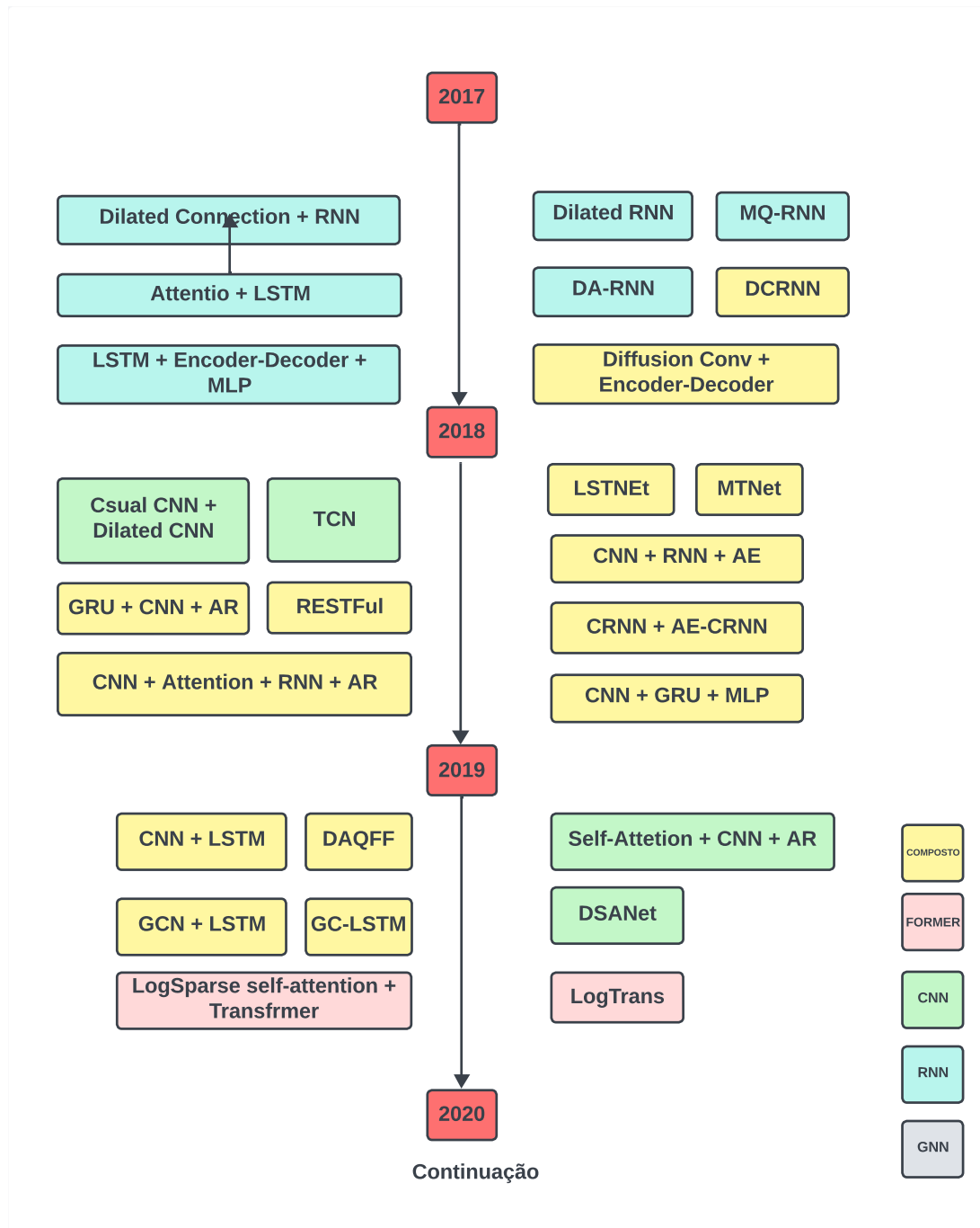
Figura 3.2: Evolução dos trabalhos em LSTF.
