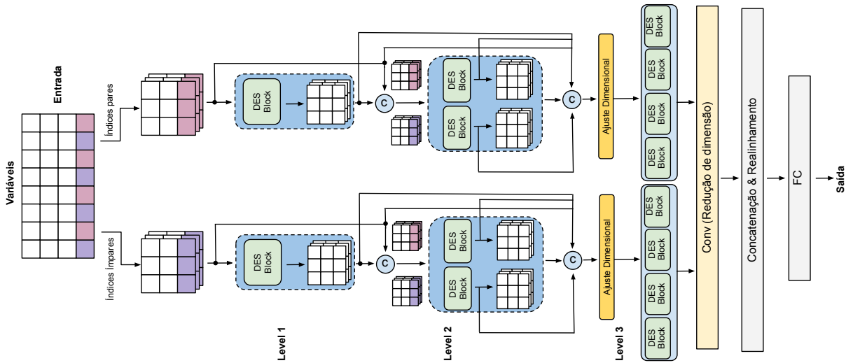
Figura 5.3: Arquitetura geral do DESCINet.
