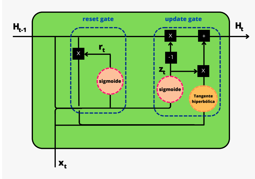
Figura 2.17: Arquitetura da Gated Recurrent Unit.
