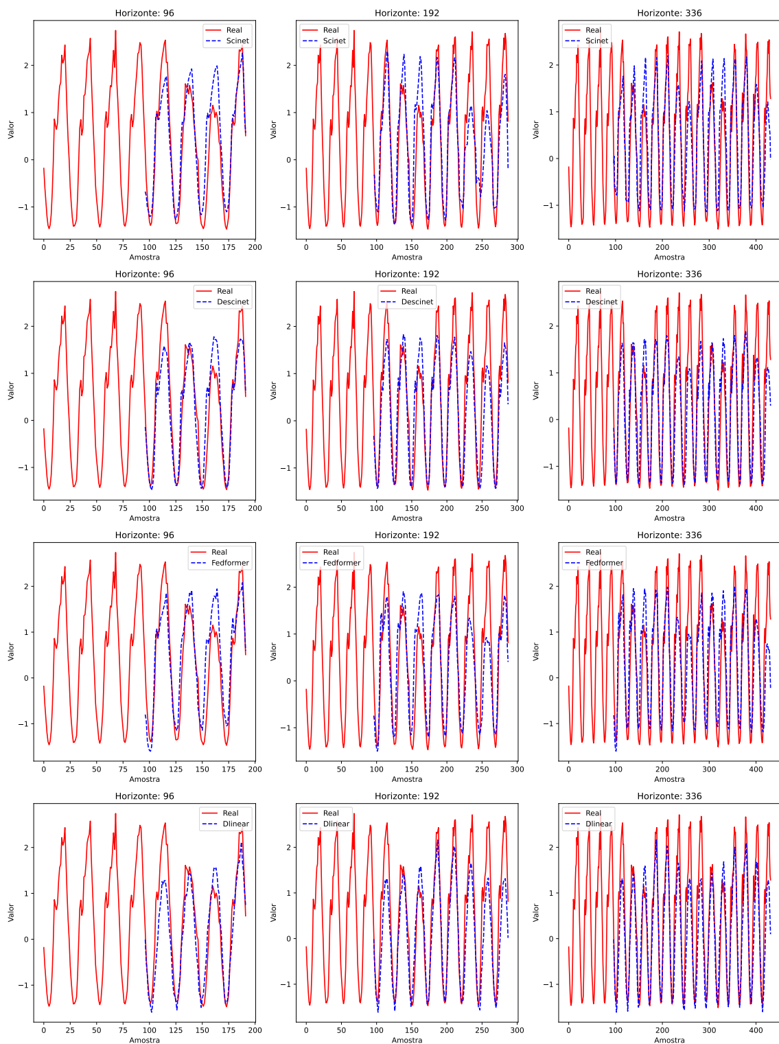
Figura 5.12: Comparativo de previsão para os horizontes de 96, 192 e 336 entre os algoritmos DESCINet, SCINet, FEDformer e DLinear no conjunto de dados multivariado Traffic .
