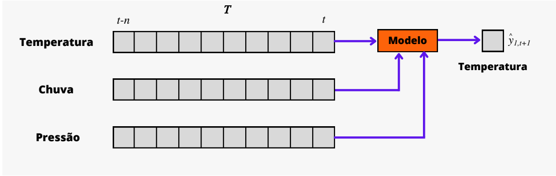
Figura 2.5: Série temporal multivariável tendo como entrada a temperatura, chuva e pressão e realizando a previsão futura da temperatura.
