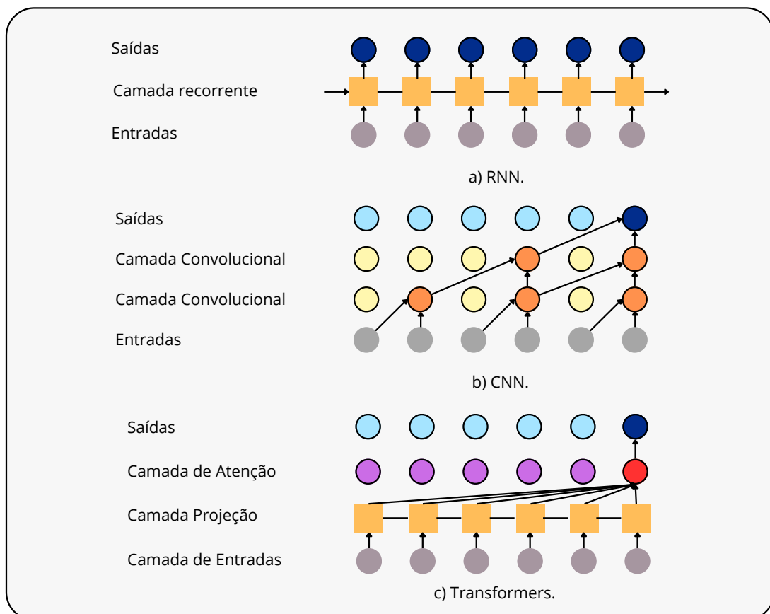
Figura 2.23: Ilustração das arquiteturas RNN, CNN e Transformers
