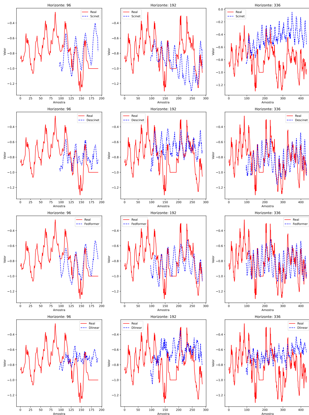
Figura 5.7: Comparativo de previsão para os horizontes de 96, 192 e 336 entre os algoritmos DESCINet, SCINet, FEDformer e DLinear no conjunto de dados multivariados ETTh1.
