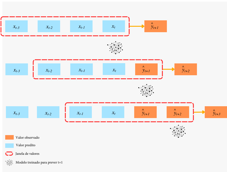
Figura 2.13: Ilustração do funcionamento do método IMS
