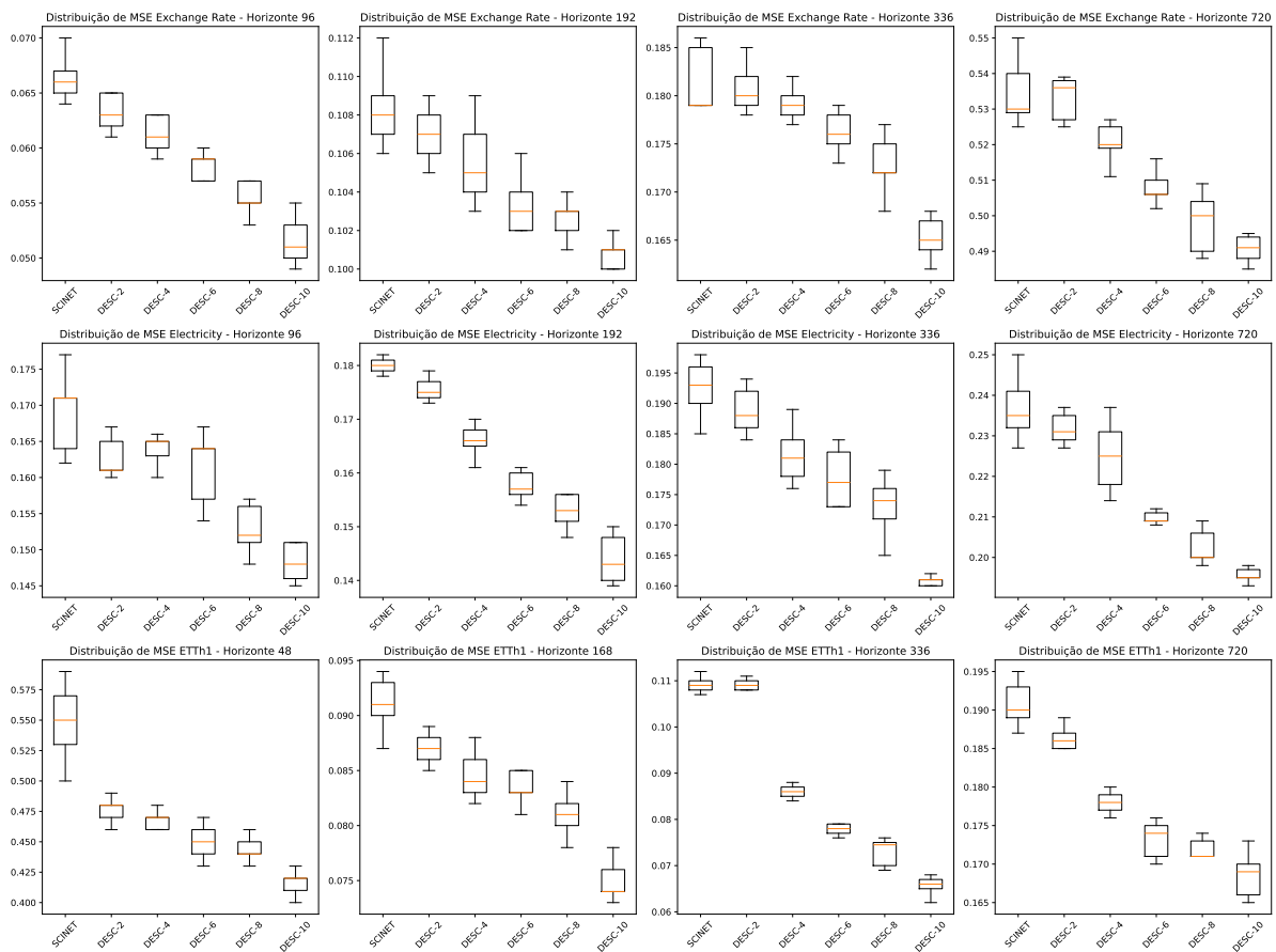
Figura 5.18: Boxplots comparando as estimativas médias do erro quadrático médio (MSE) para diferentes configurações do modelo DESCINet.
