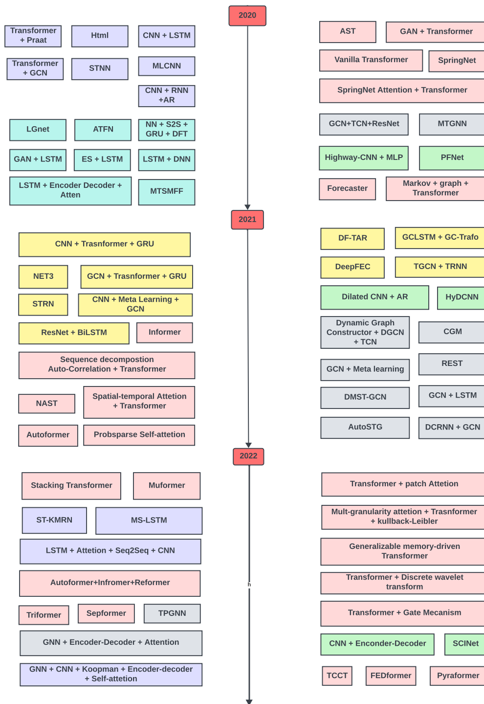
Figura 3.3: Continuação Evolução dos trabalhos em LSTF.
