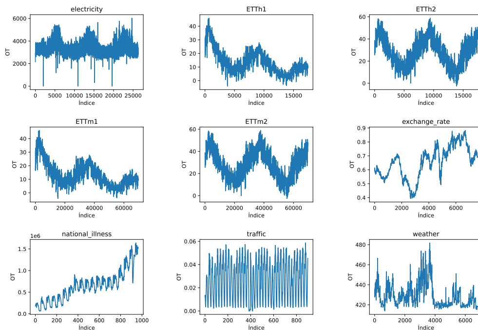
Figura 5.4: Gráfico dos conjuntos de dados utilizados para previsão.
