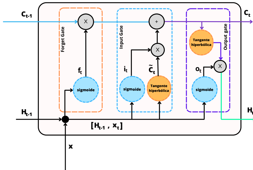
Figura 2.16: A arquitetura de um neurônio LSTM. O estado celular é representado como C , enquanto a entrada é x_t e o estado oculto é H_t .
