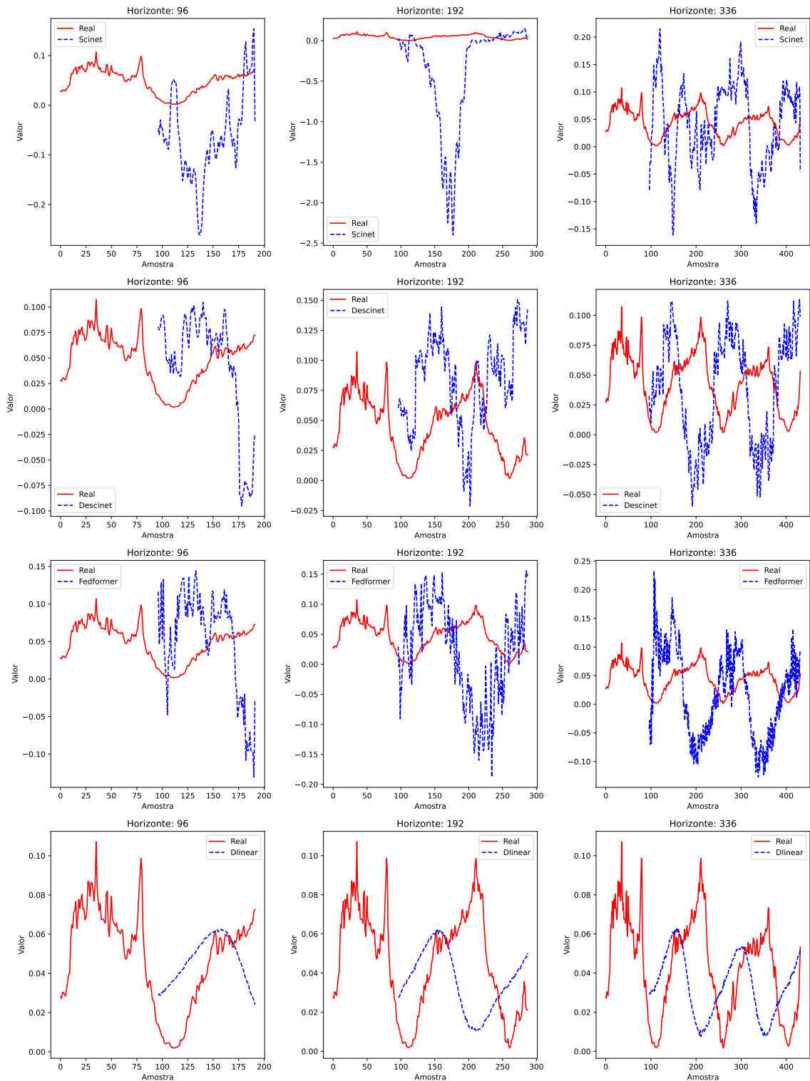
Figura 5.13: Comparativo de previsão para os horizontes de 96, 192 e 336 entre os algoritmos DESCINet, SCINet, FEDformer e DLinear no conjunto de dados multivariado Weather .
