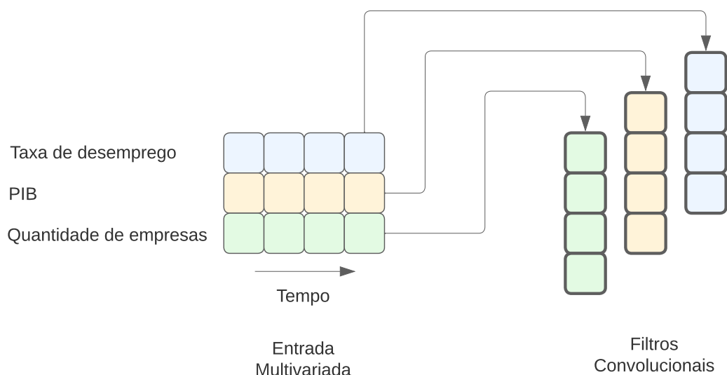
Figura 2.19: Ilustração de funcionamento de uma CNN 1D com entrada multivariada.
