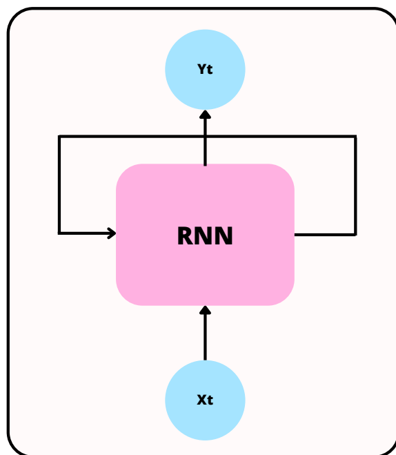
Figura 2.15: Uma representação simplificada de uma Rede Neural Recorrente mostrando como é calculado o estado oculto H_t , que é então retroalimentado na rede e combinado com a próxima entrada da sequência. Esse mecanismo permite que as RNN retenham informações de elementos anteriores da sequência e as utilizem para processar o elemento subsequente da série.
