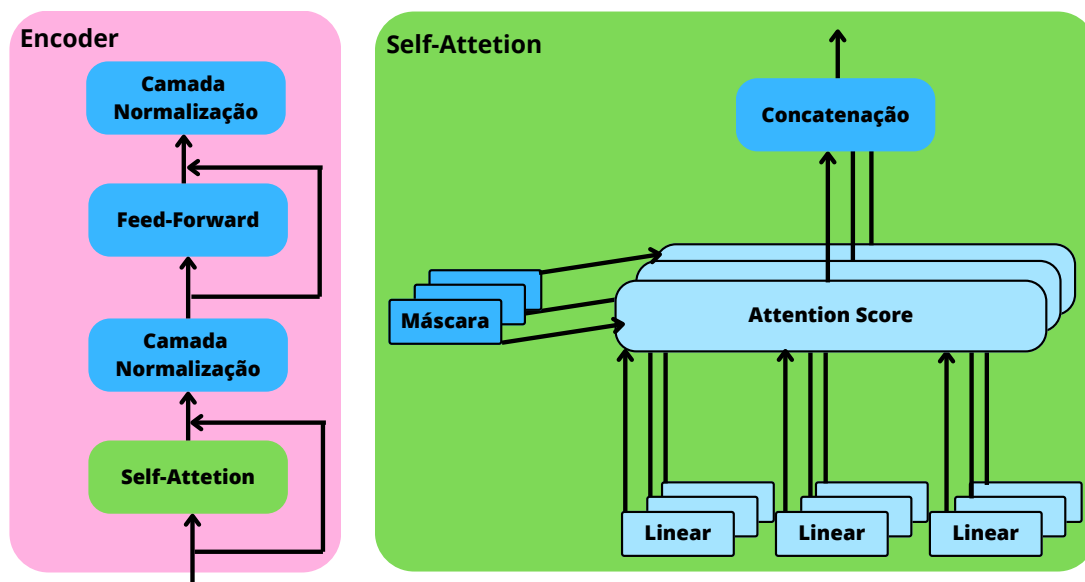
Figura 2.21: Representação da arquitetura Multi-Head Attention em um Transformer , ilustrando como o módulo de Atenção divide suas consultas (Query), chaves (Key) e valores (Value) em múltiplas cabeças de atenção. Cada cabeça processa esses elementos de forma independente, permitindo ao Transformer capturar múltiplas relações e nuances para cada palavra, e combinando-as para formar um score de atenção final.
