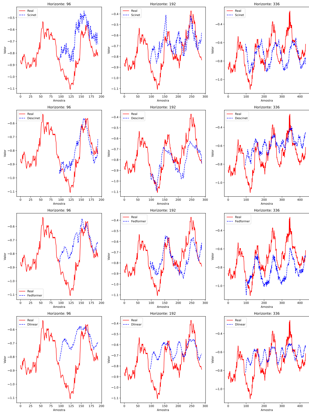
Figura 5.9: Comparativo de previsão para os horizontes de 96, 192 e 336 entre os algoritmos DESCINet, SCINet, FEDformer e DLinear no conjunto de dados multivariados ETTm1.
