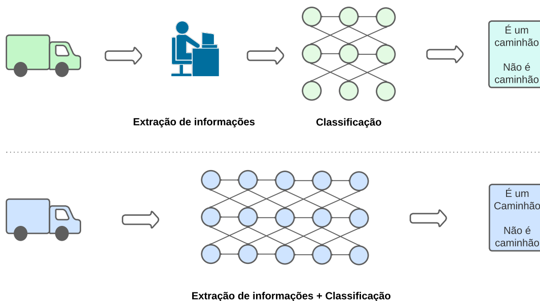
Figura 2.14: Diagrama comparativo entre aprendizado de máquina tradicional e aprendizado profundo, destacando a automação na extração de características por redes neurais profundas no aprendizado profundo.
