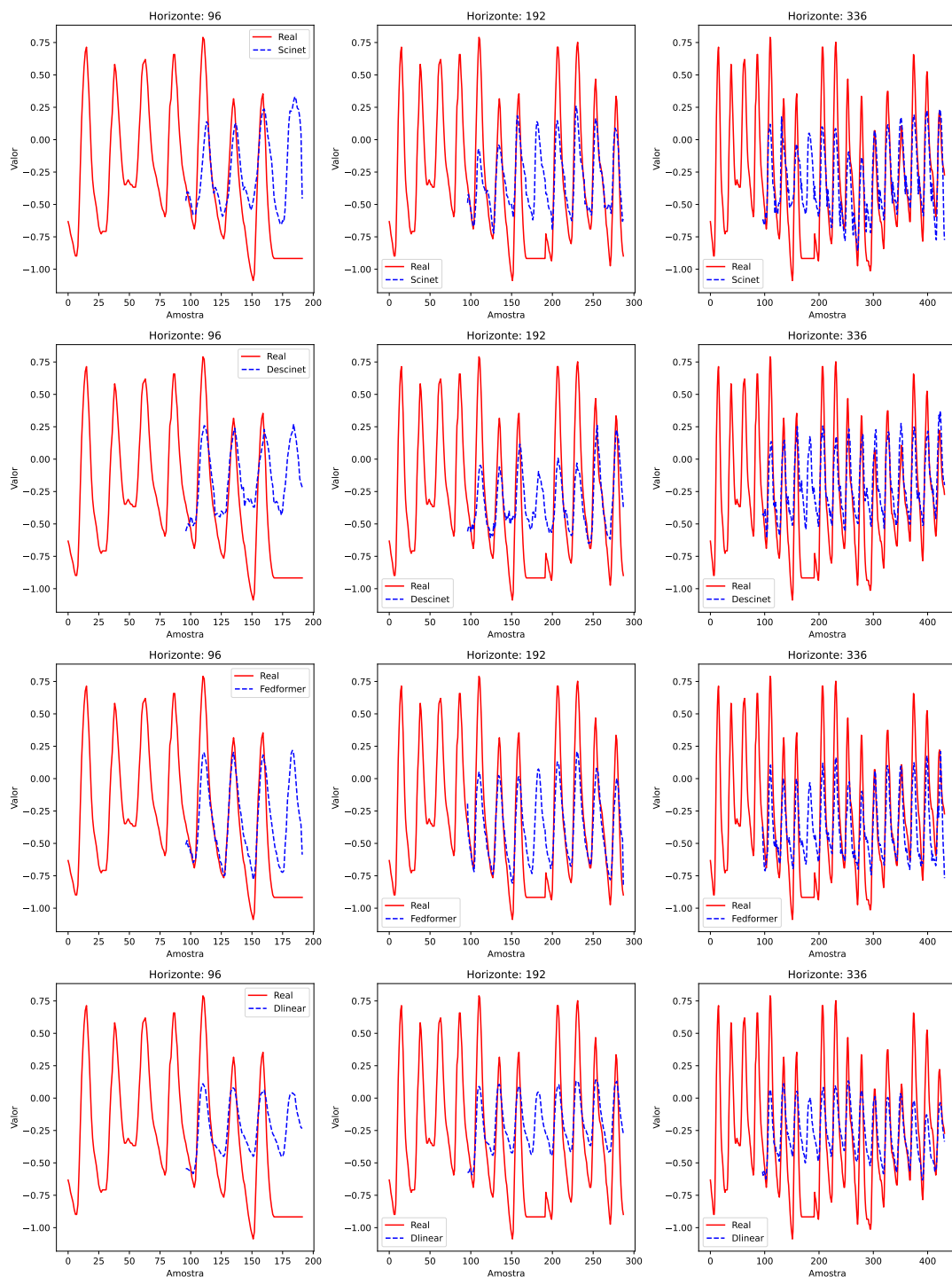
Figura 5.8: Comparativo de previsão para os horizontes de 96, 192 e 336 entre os algoritmos DESCINet, SCINet, FEDformer e DLinear no conjunto de dados multivariados ETTh2.
