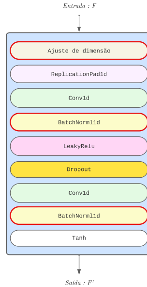
Figura 5.1: Arquitetura geral do DESBlock. Fonte: Autoria própria.
