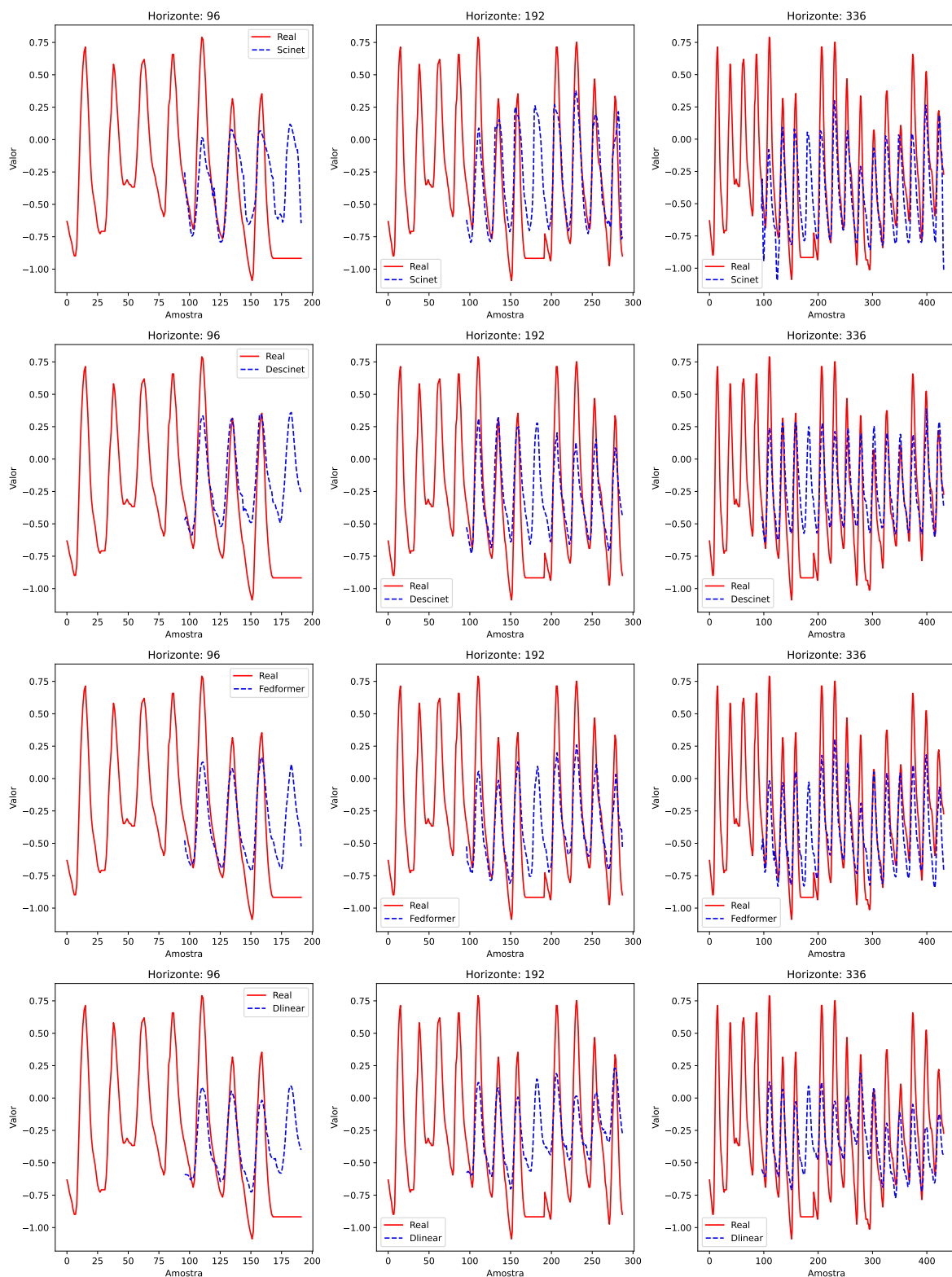
Figura 5.6: Comparativo de previsão para os horizontes de 96, 192 e 336 entre os algoritmos DESCINet, SCINet, FEDformer e DLinear no conjunto de dados univariado ETTh2.
