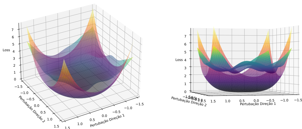
Figura 5.15: Comparativo de loss landscape entre SCINet e DESCINet.
