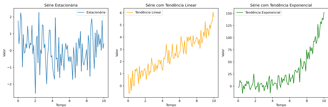
Figura 2.9: a) Série temporal estacionária. b) Série temporal não-estacionária com tendência linear. c) Série temporal não-estacionária com crescimento exponencial.
