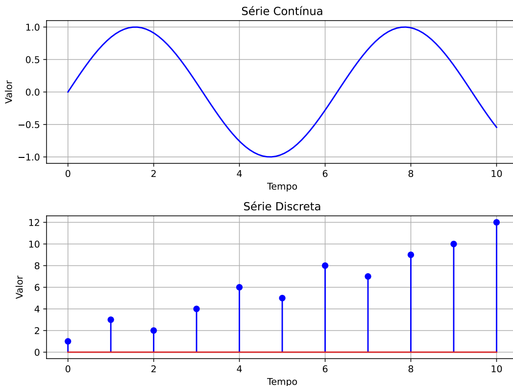
Figura 2.3: Série temporal apresentada em dois formatos distintos: contínuo e discreto, respectivamente
