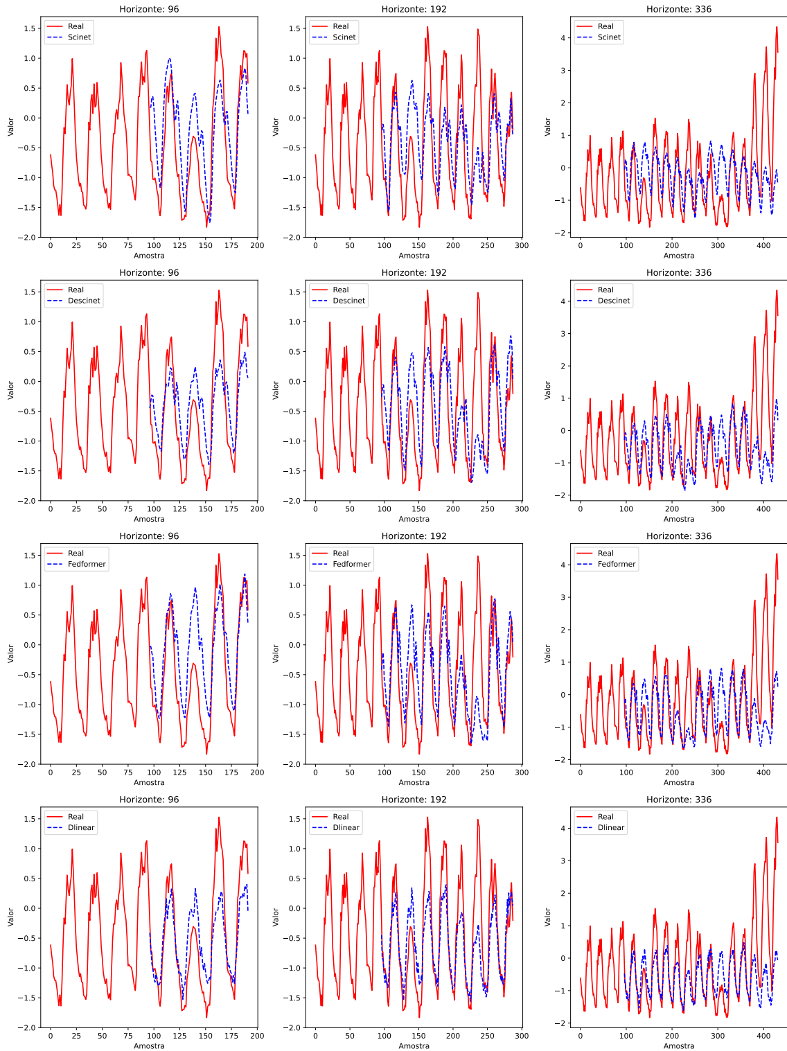
Figura 5.11: Comparativo de previsão para os horizontes de 96, 192 e 336 entre os algoritmos DESCINet, SCINet, FEDformer e DLinear no conjunto de dados multivariado Electricity .
