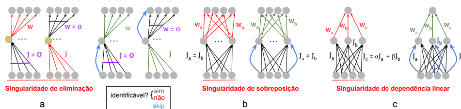
Figura 4.4: Singularidades em uma camada totalmente conectada e como pular conexões evita isso. Adaptado de Orhan (2017).
