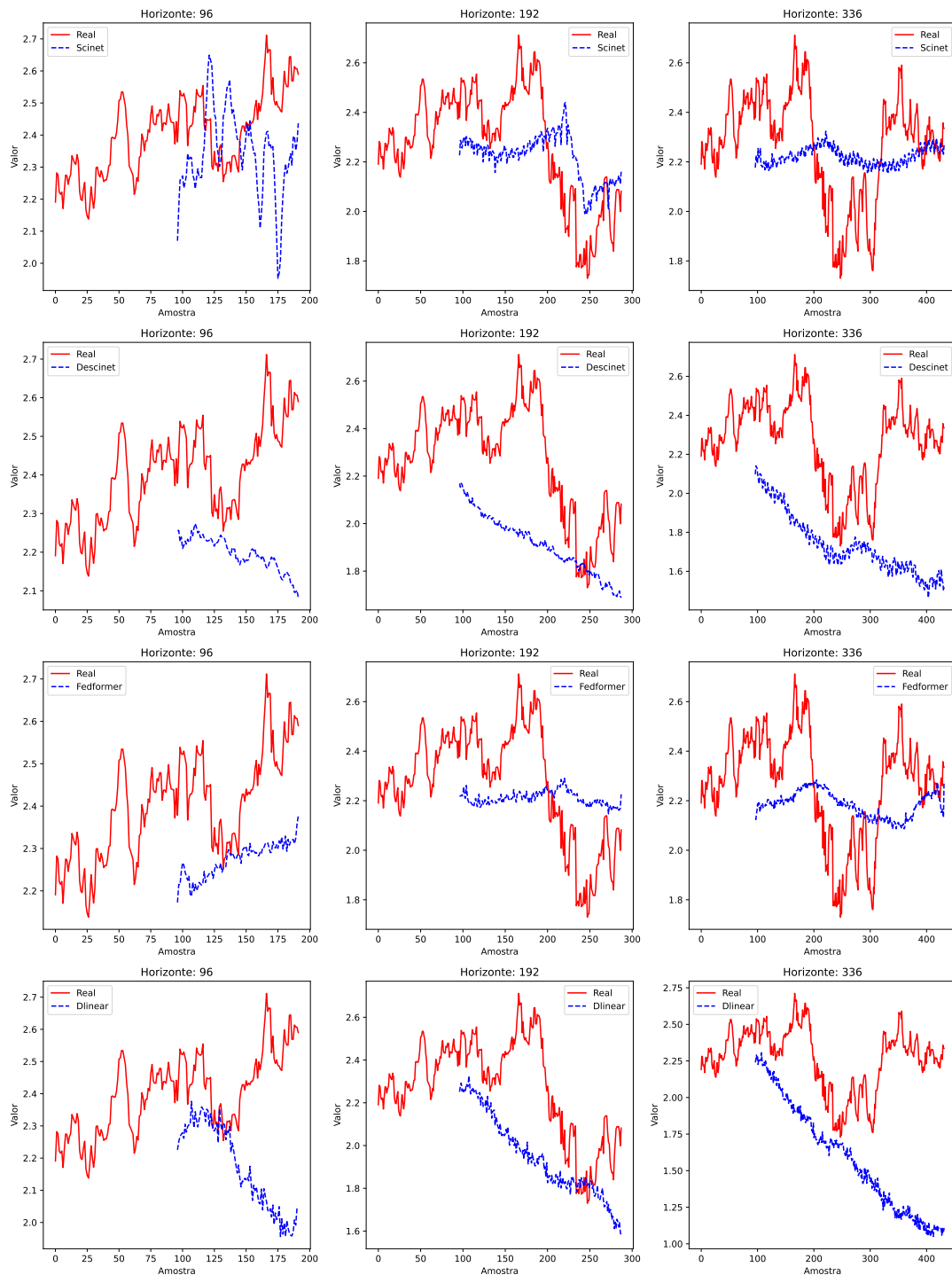
Figura 5.10: Comparativo de previsão para os horizontes de 96, 192 e 336 entre os algoritmos DESCINet, SCINet, FEDformer e DLinear no conjunto de dados multivariado Exchange Rate .
