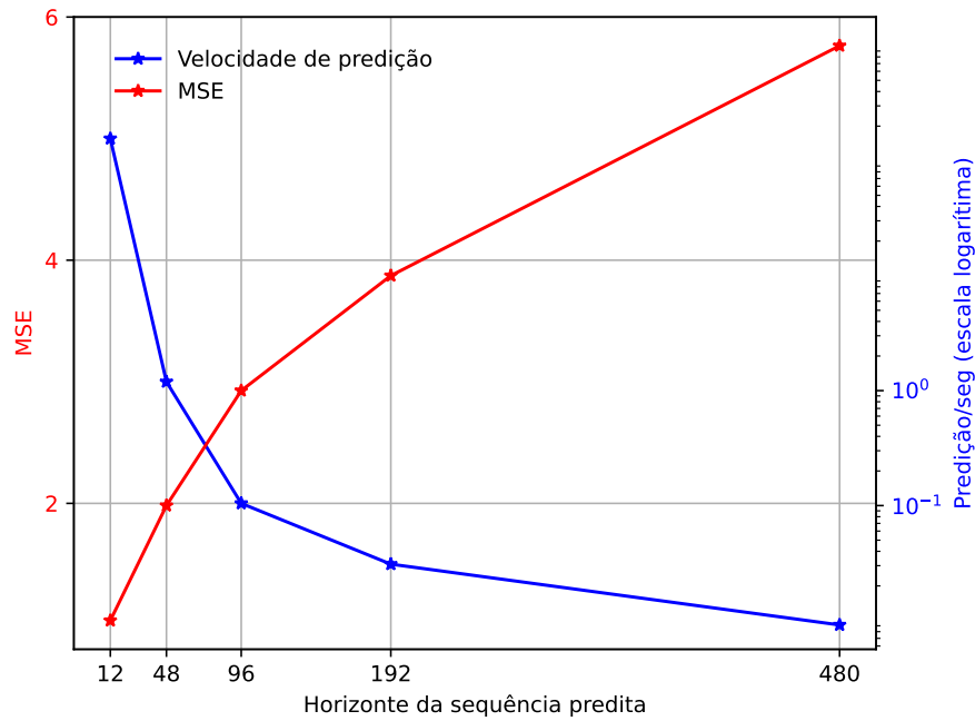
Figura 2.11: A capacidade de previsão de uma LSTM na previsão a longo prazo (STL). A partir de um comprimento de 48, o MSE aumenta e a velocidade de inferência cai rapidamente.
