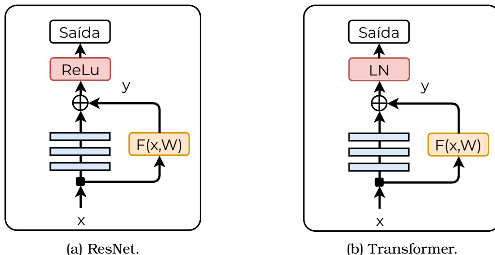
Figura 4.3: Representação da conexão residual: (a) Unidade Residual Convencional (He et al., 2016), (b) Unidade Residual em Transformers (LN = Normalização de Camadas) (Vaswani et al., 2017a). Adaptado de Liu et al. (2020) .
