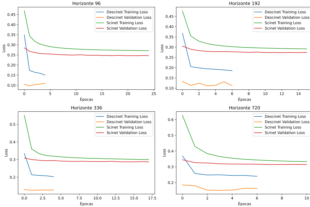
Figura 5.16: Comparativo de loss de treino e validação entre SCINet e DESCINet utilizando o conjunto de dados ETTh1.
