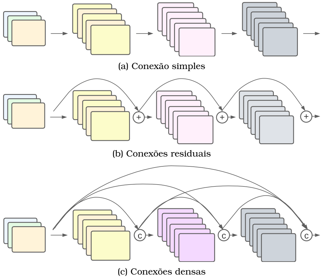
Figura 4.2: Ilustração das diferentes arquiteturas de conexões em redes neurais: (a) apresenta uma arquitetura de conexão simples, (b) exibe conexões residuais, e (c) mostra conexões densas.
