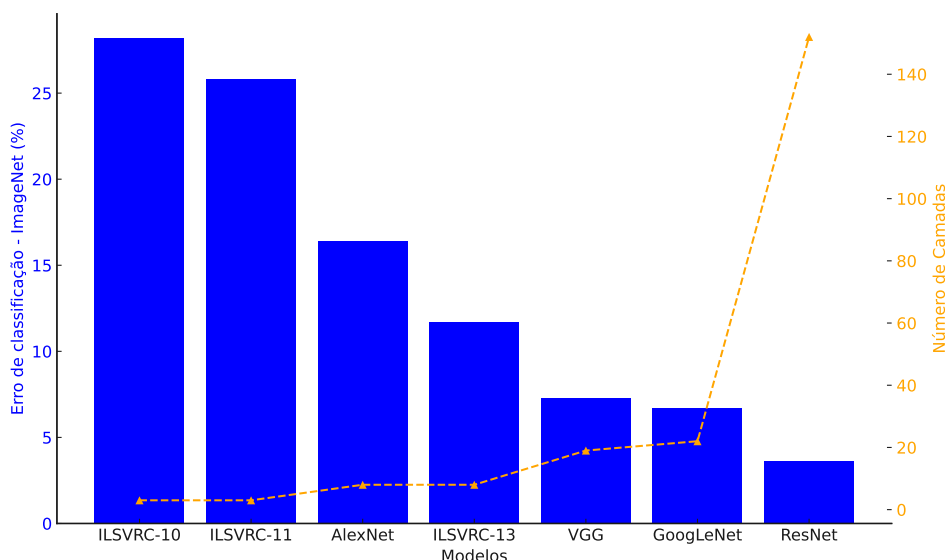
Figura 4.1: Evolução da quantidade de camadas em modelos neurais.
