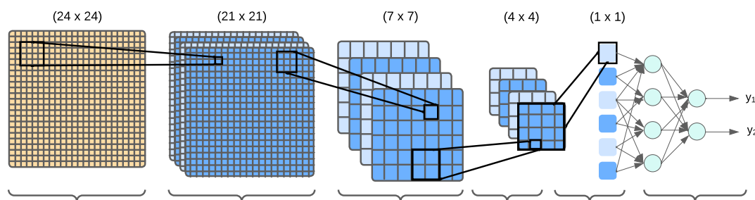
Figura 2.18: A ilustração de uma amostra de CNN com 2 camadas de convolução e uma camada totalmente conectada.
