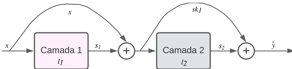
Figura 4.6: Ilustração de rede sem conexões residuais.
