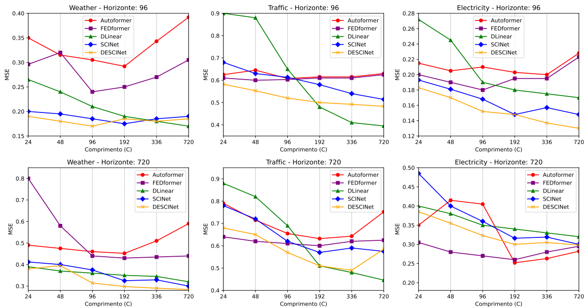
Figura 5.17: Desempenho de previsão (MSE) com janelas de observação variáveis nos 3 maiores conjuntos de dados: Traffic , Electricity e Weather . As janelas de observação são selecionadas para serem L = 24, 48, 96, 192, 336, 720 , e os horizontes de previsão são T = 96, 720 .
