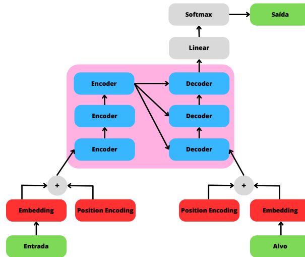
Figura 2.20: Representação esquemática da arquitetura do Transformer mostrando o componente de codificação ( encoders ) e o componente de decodificação ( decoders ). A transformação da entrada é ilustrada, com as setas indicando o fluxo de dados do modelo até a saída.
