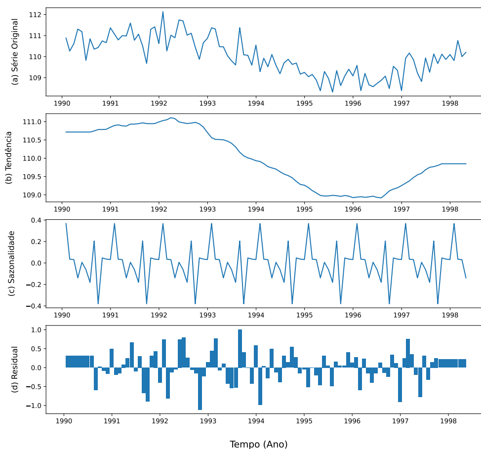
Figura 2.7: Componentes extraídos da série temporal de uma série gerada sinteticamente.
