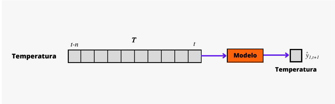
Figura 2.4: Série temporal com única entrada e realizando a previsão futura desta variável.
