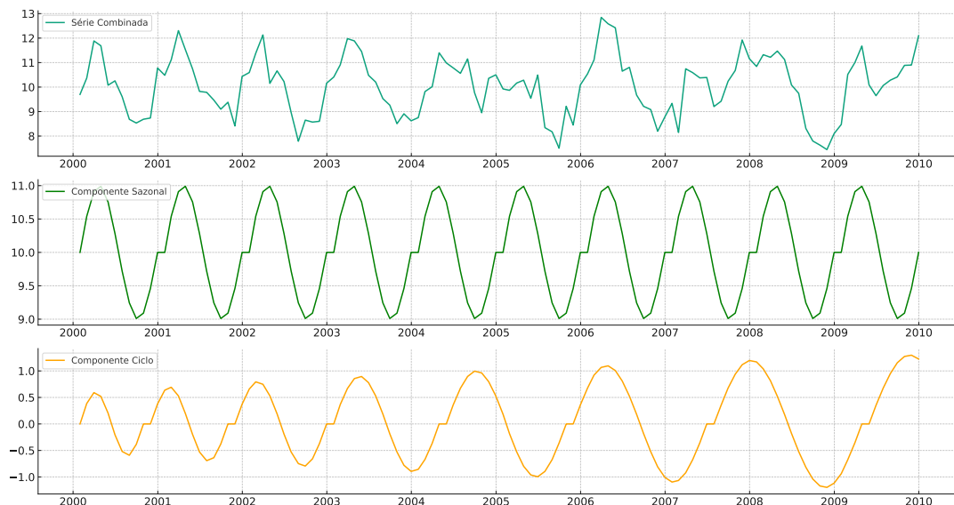
Figura 2.8: Exemplo comparativo de variação de ciclo e sazonalidade .
