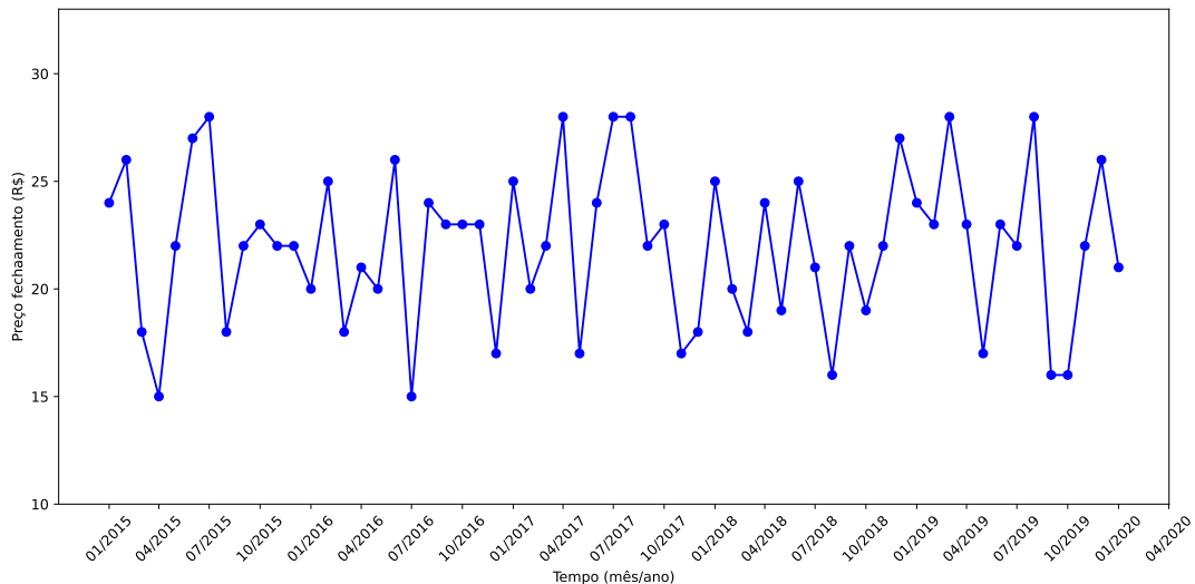
Figura 2.2: Série temporal irregular.
