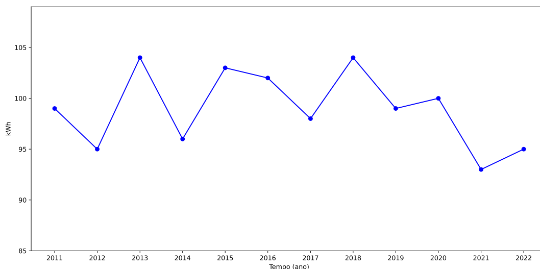
Figura 2.1: Série temporal fictícia do consumo de energia de uma casa.
