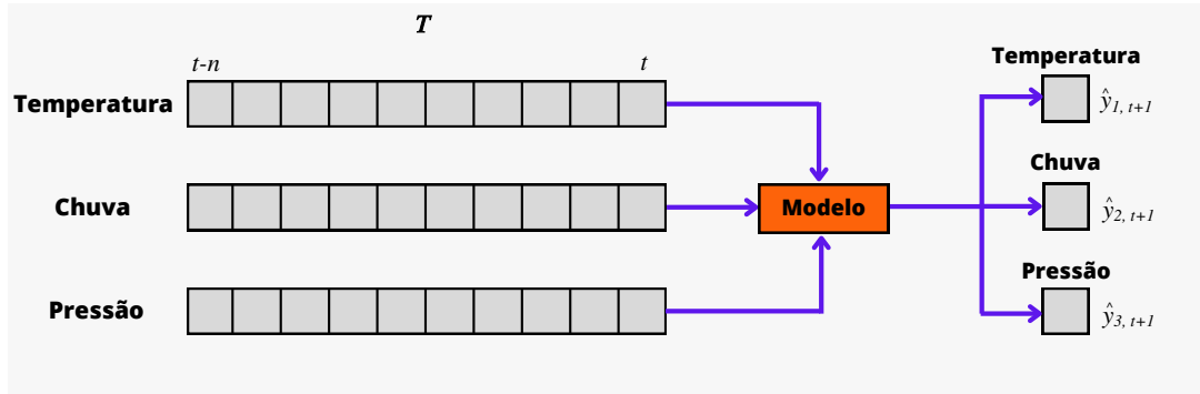
Figura 2.6: Série temporal tendo como entrada a temperatura, chuva e pressão e realizando a previsão futura da temperatura, chuva e pressão..
