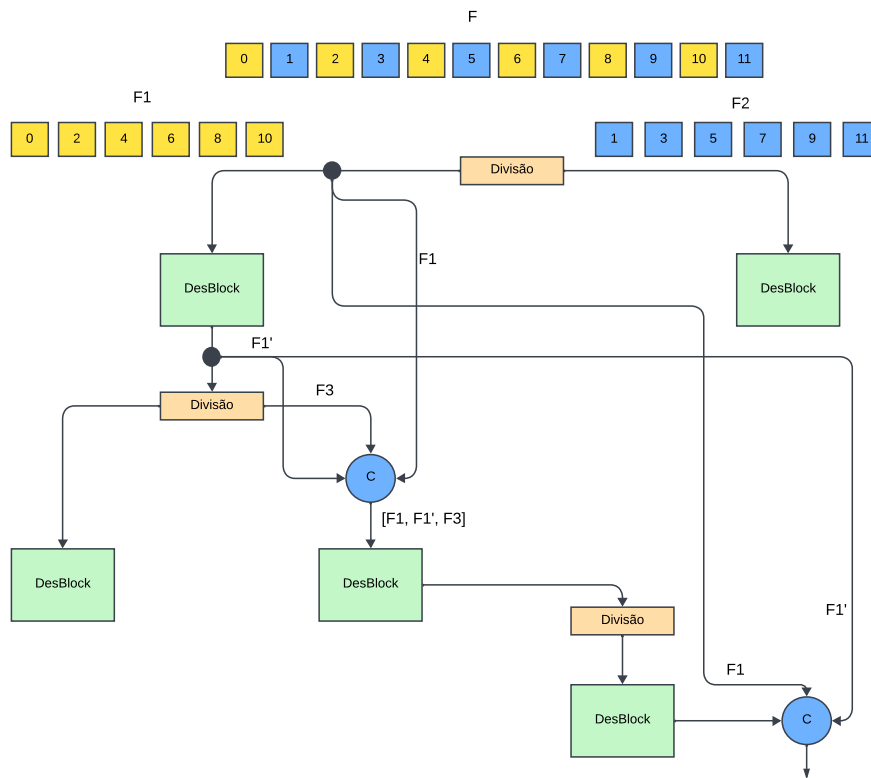
Figura 5.2: Passo a passo do fluxo de informações através do modelo DESCINet.
