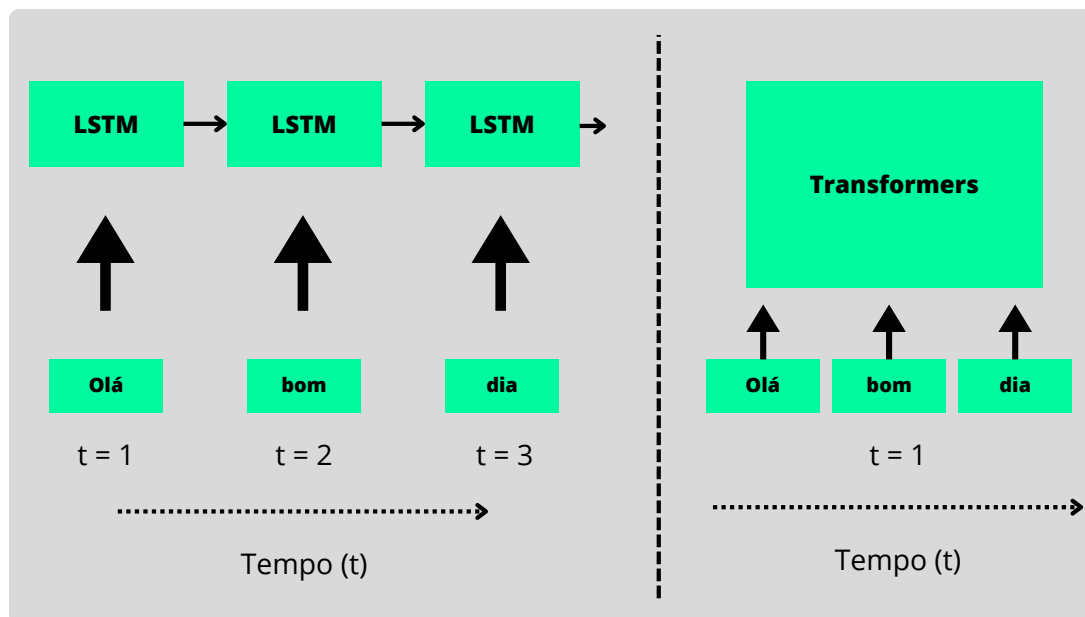
Figura 2.22: Comparativo entre RNN e Transformers
