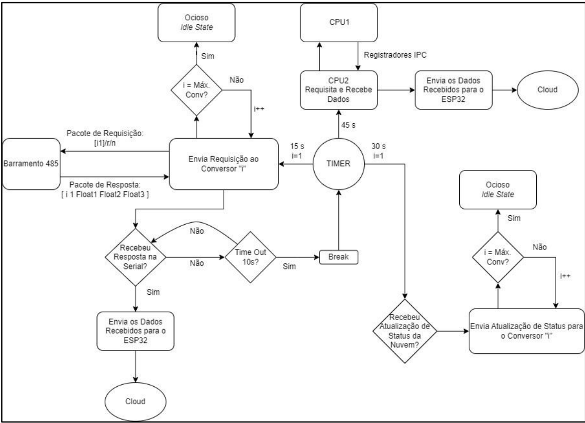
Figura 25. Fluxo de Comunicação do Sistema.
