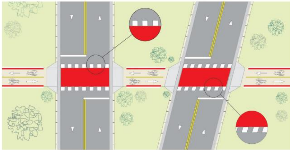
Figura 11 - Marcação de Cruzamentos rodociclovitários.
