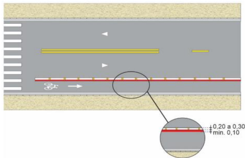
Figura 9 – Modelo de marcação de ciclofaixa ao longo da via.
