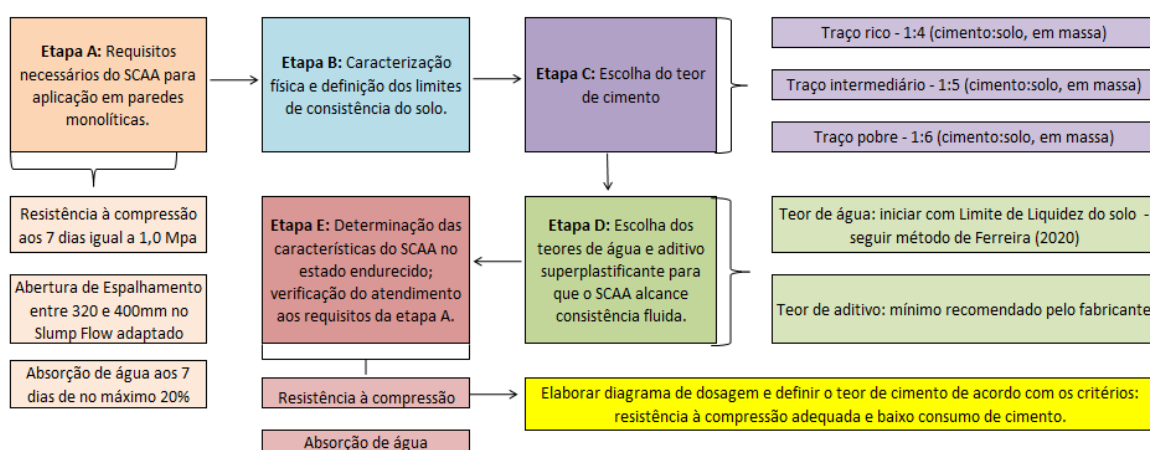
Figura 20. Metodologia de dosagem para SCAA
