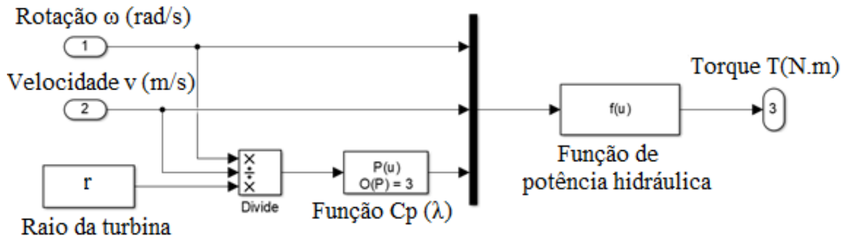
Figura 14 – Subsistema para a simulação da turbina em regime permanente.
