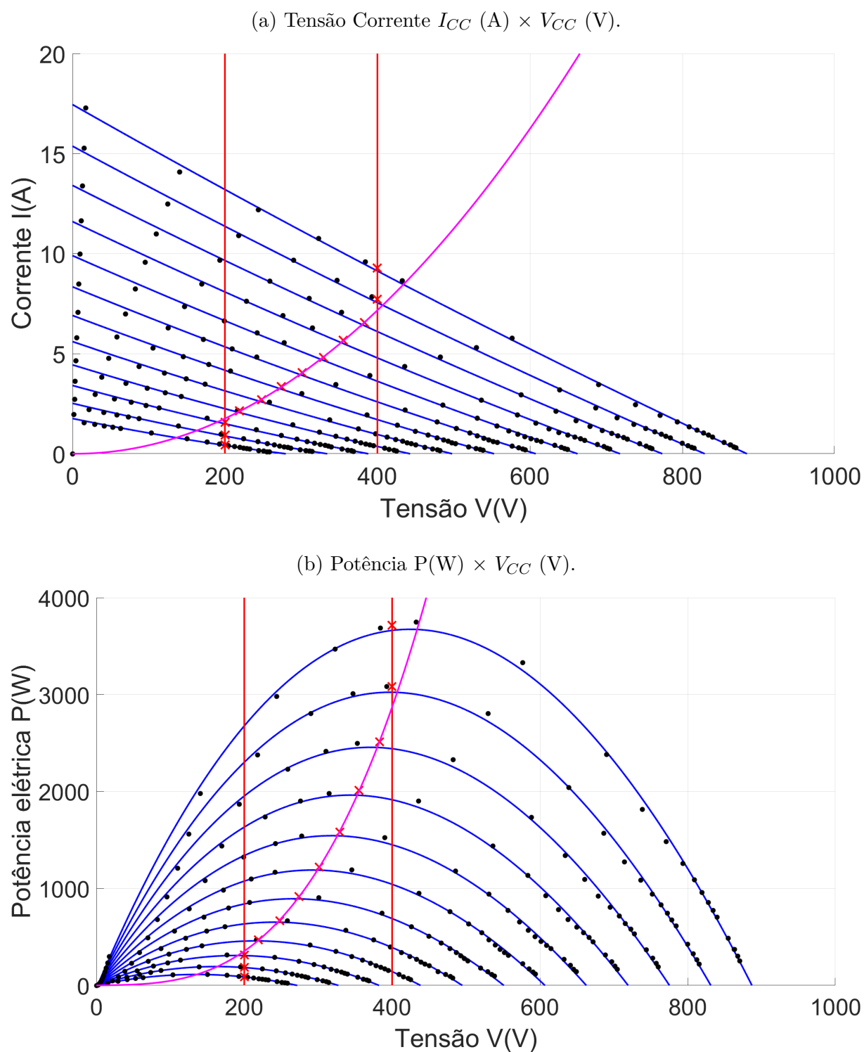
Figura 35 – Curvas características de operação do sistema com a turbina de eixo horizontal.
