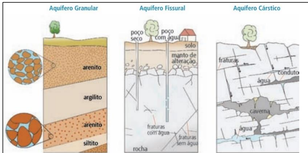
Figura 2 - Classificação dos aquíferos a partir do tipo de porosidade da rocha
