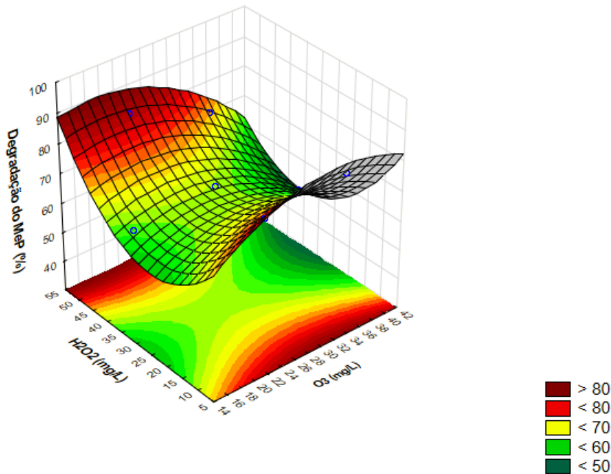
Figura 13 - Gráfico de superfície de resposta da interação entre [O_3] e [H_2O_2] na % de degradação do MeP
