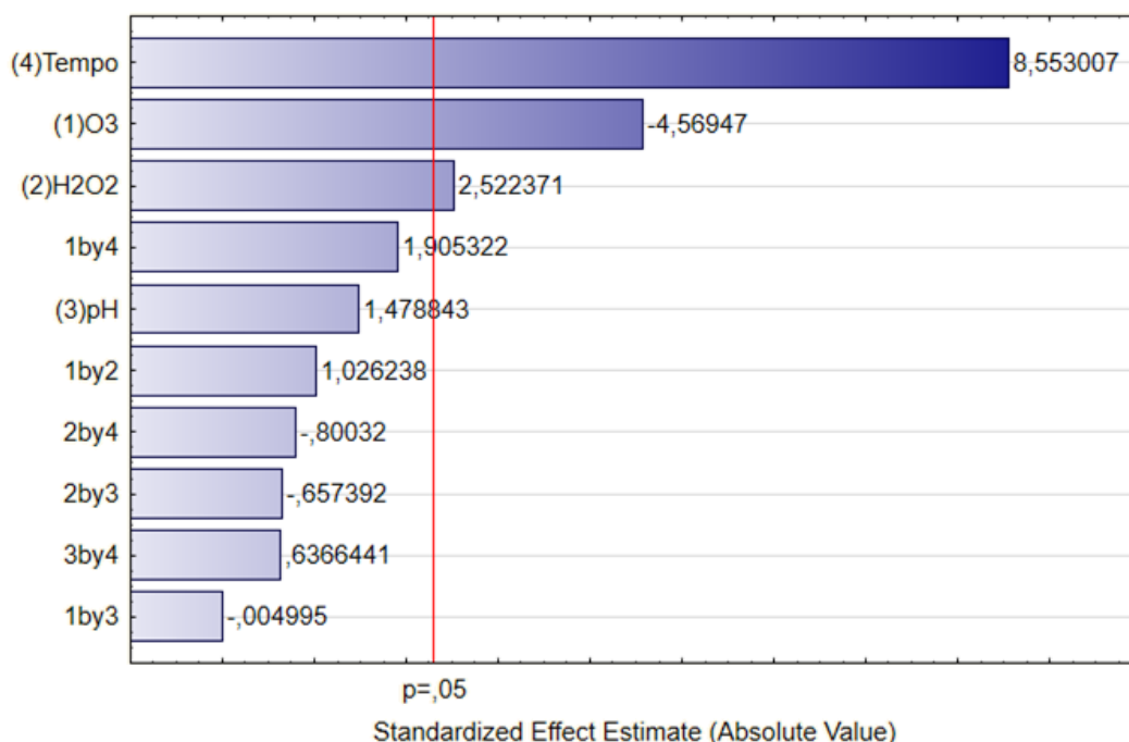
Figura 6 - Gráfico de Pareto dos valores do efeito de cada variável e a interação entre elas com relação à degradação do MeP, com base nos experimentos do planejamento fatorial
