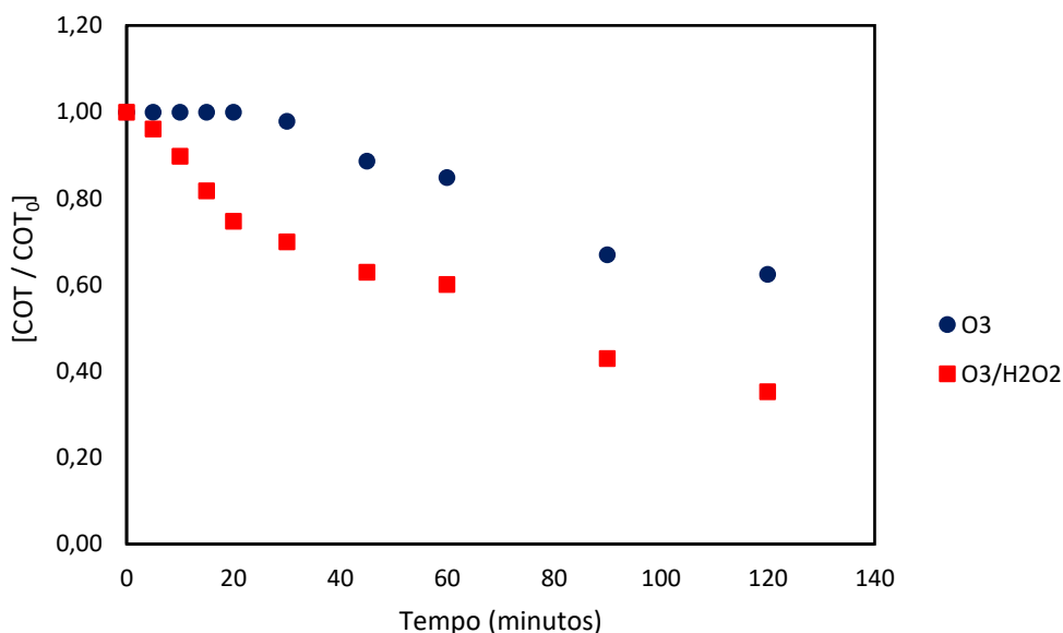
Figura 7 - Gráfico do decaimento de carbono orgânico total para os processos de O_3 e O_3/H_2O_2 sob as mesmas condições: 41 \text{ mg/L} de O_3 ; adição de 60 \text{ mg/L} de H_2O_2 e pH do efluente igual a 7,0 \pm 0,2
