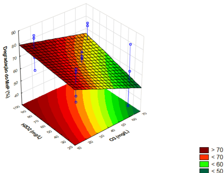
Figura 9 - Gráfico de superfície de resposta da interação entre [O_3] e [H_2O_2] na % degradação do MeP
