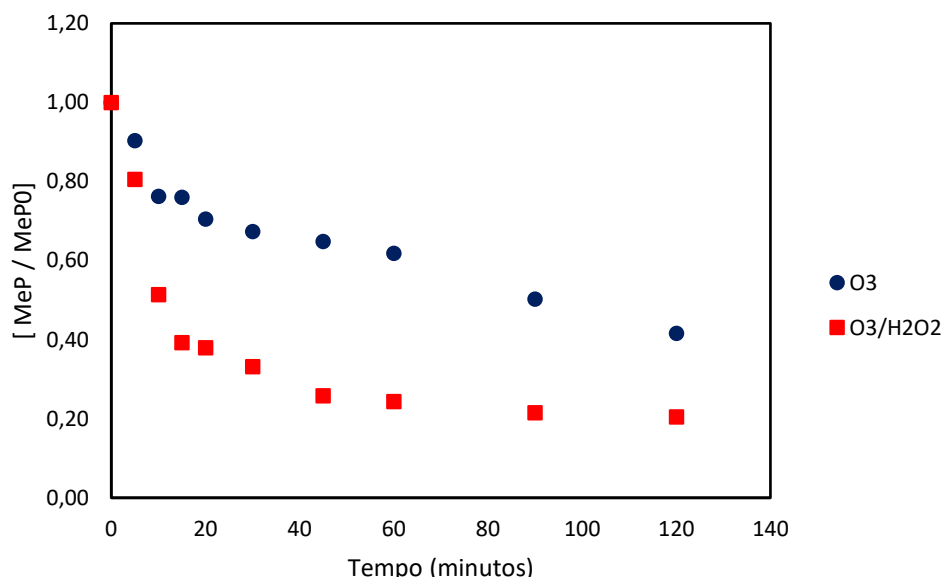
Figura 8- Gráfico do decaimento da concentração de MeP para os processos de O_3 e O_3/H_2O_2 sob as mesmas condições: 41 mg/L de O_3 ; adição de 60 mg/L de H_2O_2 e pH do efluente igual a 7,0 \pm 0,2
