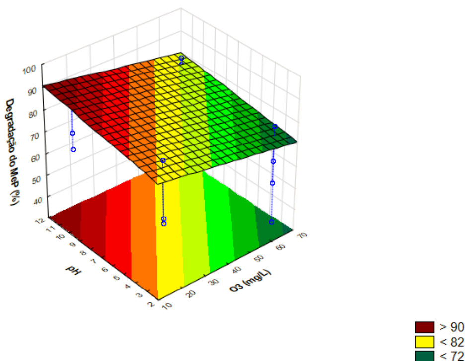
Figura 10 - Gráfico de superfície de resposta da interação entre o pH da solução e a [O_3] na % de degradação do MeP
