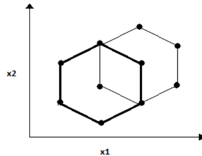
Figura 2 - Design de um planejamento de Doehlert para duas variáveis
