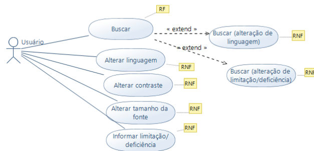
Figura 5.2: Diagrama de casos de uso do buscador
