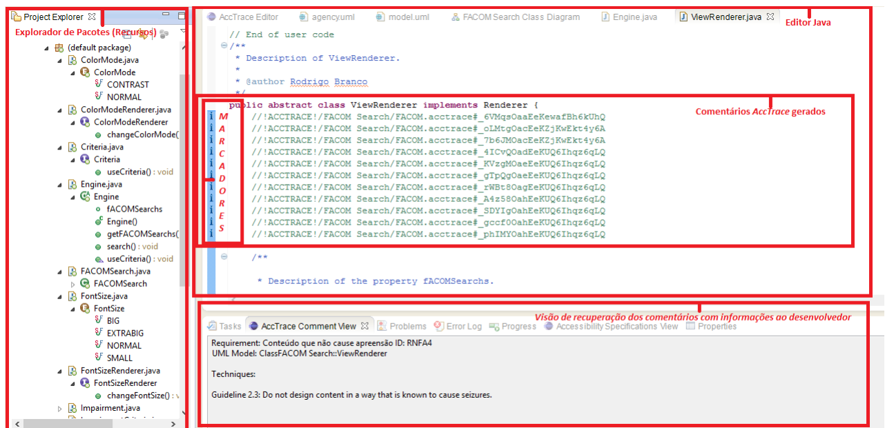
Figura 5.9: Visualização do código gerado, com os comentários AccTrace personalizados
