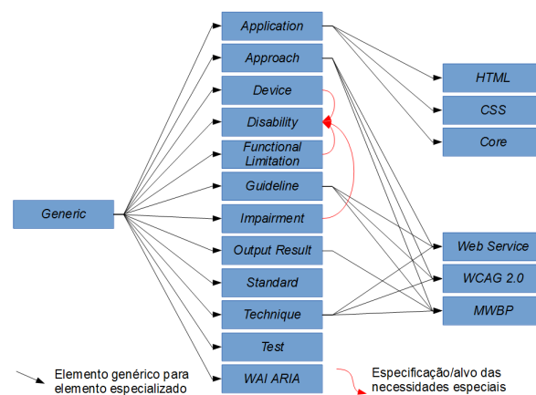
Figura 4.14: Relacionamento entre os elementos da ontologia (Elementos retirados da ontologia)
