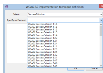
Figura 4.16: Elementos disponíveis para a ontologia SuccessCriterion
