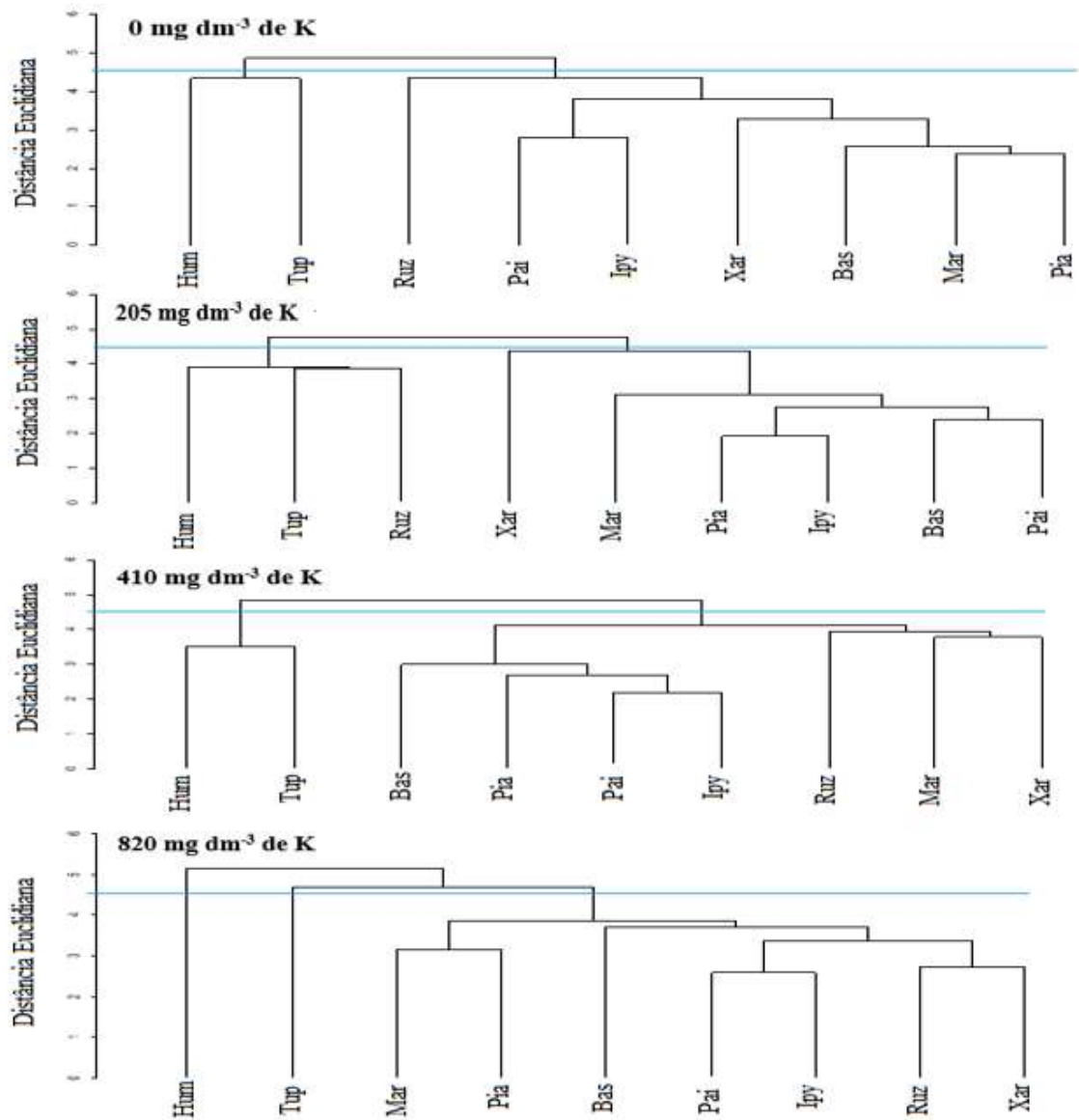
FIGURA 1 Dendrograma de agrupamento de cultivares de Brachiaria em função das características morfológicas, estruturais e densidade de perfilhos nas diferentes doses de potássio avaliadas. Hum – Brachiaria humidicula cv. Comum; Tup – cultivar Tupi; Ruz – cultivar Ruziziensis; Xar – cultivar Xaraés; Mar – cultivar Marandu; Pia – cultivar Piatã; Ipy – Cultivar BRS Ipyporã; Bas – Cultivar Basilisk; Pai – cultivar Paiaguás.
