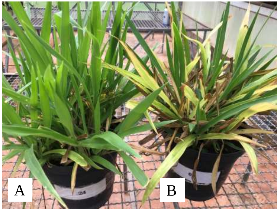
Figura 3 - Sintoma de mancha foliar ( Bipolaris maydis ), em função do fornecimento de 205 mg dm -3 de potássio (A) e da ausência de adubação (B) na cultivar Ipyporã (híbrido B. ruziziensis e B. brizantha ).
