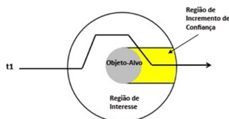
Figura 3.11: Exemplo de uma trajetória que passa pela região de incremento de confiança.
